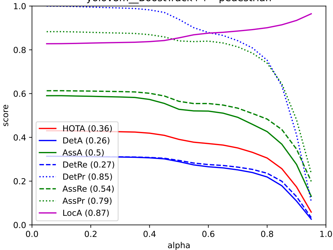
yolov8m_BoostTrack++ - pedestrian
