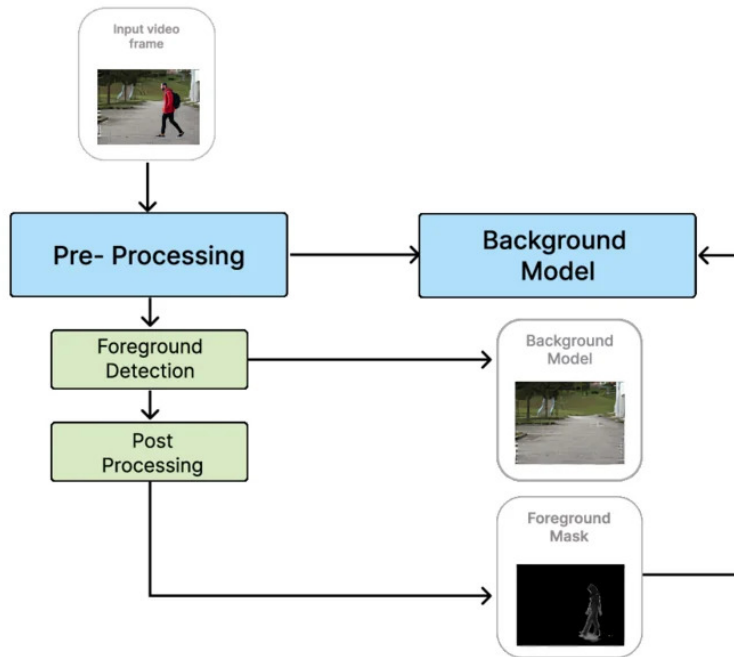
Rysunek 1. Wizualizacja procesu odejmowania tła. Źródło: [55]
