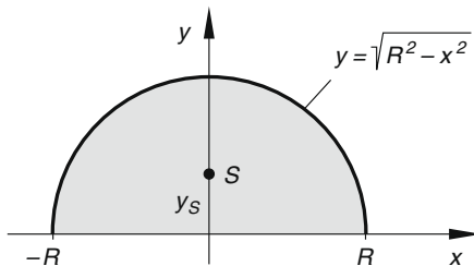
Bild V-83 Zur Berechnung der Schwerpunktskoordinaten einer homogenen Halbkreisfläche
