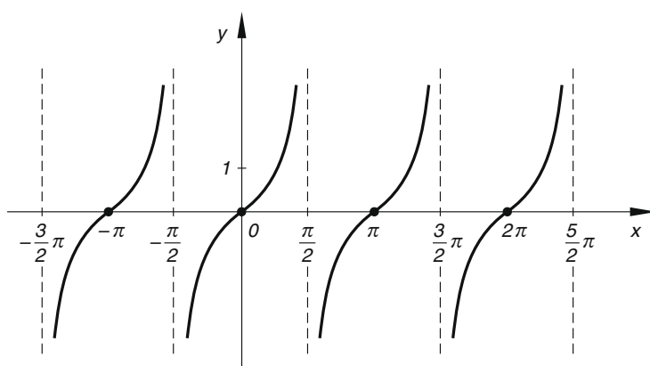
Bild III-113 Funktionsgraph der Tangensfunktion
