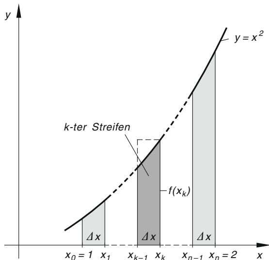
Bild V-10 Zur Berechnung des bestimmten Integrals \int_1^2 x^2 dx als Grenzwert der Obersumme
