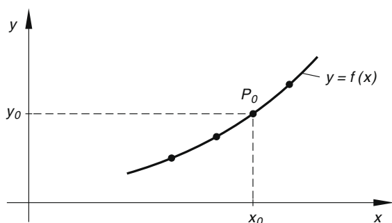
Bild III-1 Graph einer Funktion
