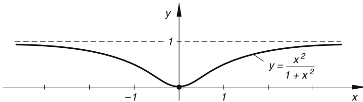
Bild IV-39 Funktionsgraph von y = \frac{x^2}{1+x^2}
