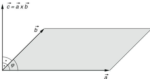
Bild II-51 Zum Begriff des Vektorsproduktes zweier Vektoren
