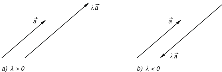
Bild II-17 Zur Multiplikation eines Vektors \vec{a} mit einem Skalar \lambda
