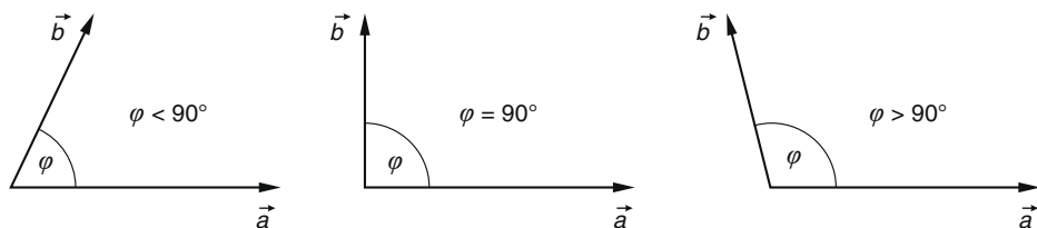
Bild II-30 Winkel zwischen zwei vom Nullvektor verschiedenen Vektoren
