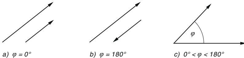
Bild II-33 a) und b) Kollineare Vektoren c) Nichtkollineare Vektoren
