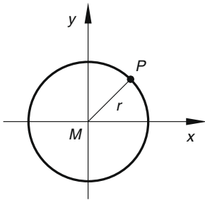
Bild III-90 Mittelpunktskreis
