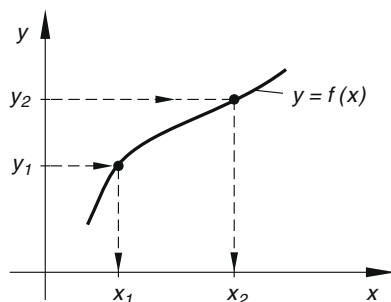
Bild III-26 Zur Umkehrung einer Funktion
