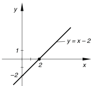
Bild III-7 Einfache Nullstelle
