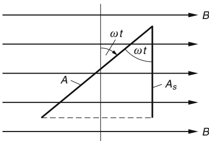
Bild IV-16 Zum Induktionsgesetz
