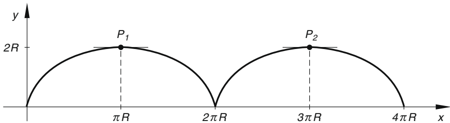
Bild IV-8 Gewöhnliche Zykloide (Rollkurve)
