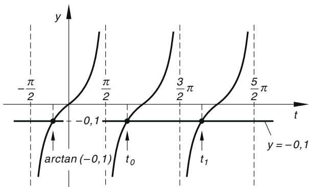
Bild IV-57 Positive Lösungen der Gleichung \tan t = -0,1 (Skizze)
