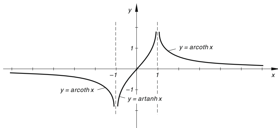
Bild III-172 Funktionsgraphen der Areafunktionen y = \operatorname{artanh} x und y = \operatorname{arcoth} x
