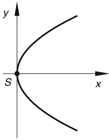
Bild III-99 Zur Scheitelgleichung der Parabel
