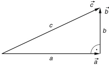
Bild II-45 Zur Herleitung des Satzes des Pythagoras
