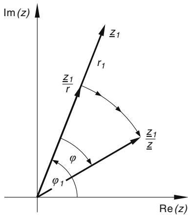
Bild VII-27 Zur Division zweier komplexer Zahlen
