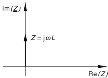
Bild VII-43 Induktiver Blindwiderstand
