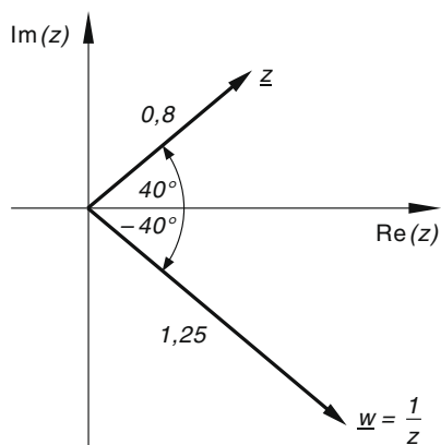
Bild VII-59 Inversion der komplexen Zahl z = 0,8 \cdot e^{j40^\circ}
