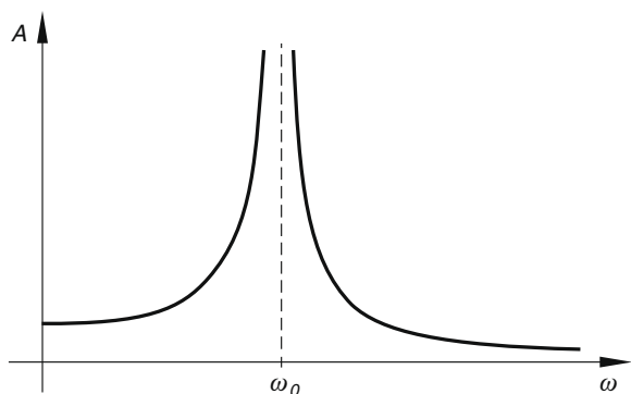
Bild III-50 Resonanzkurve bei einer erzwungenen mechanischen Schwingung
