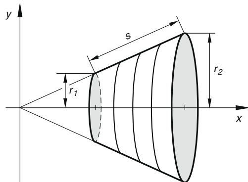
Bild V-65 Kegelstumpf
