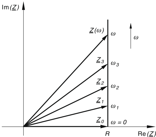
Bild VII-49 Widerstands Ortskurve der Reihenschaltung aus Bild VII-48
