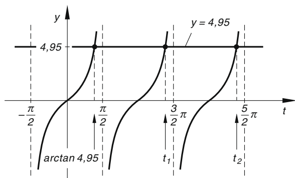
Bild IV-58 Positive Lösungen der Gleichung \tan t = 4,95 (Skizze)
