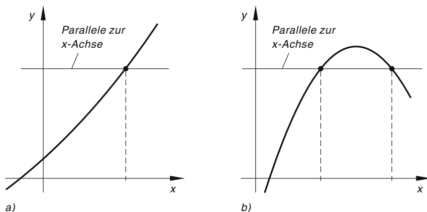
Bild III-28 Zur Umkehrung einer Funktion
