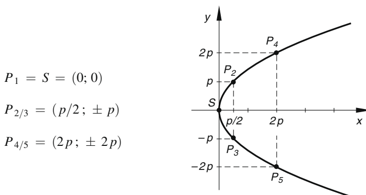
Bild III-101 Zur Konstruktion einer Parabel aus 5 Punkten
