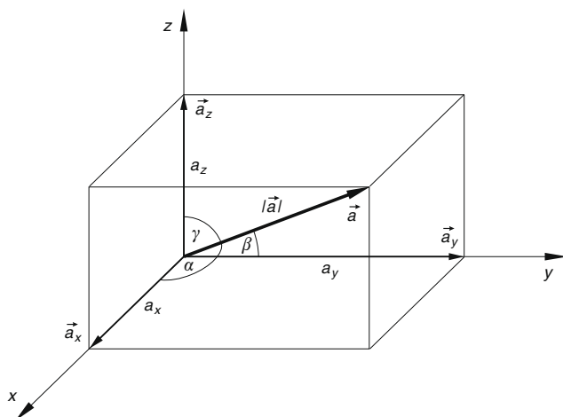
Bild II-46 Richtungswinkel eines Vektors
