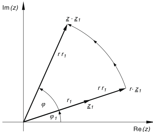
Bild VII-26 Zur Multiplikation zweier komplexer Zahlen
