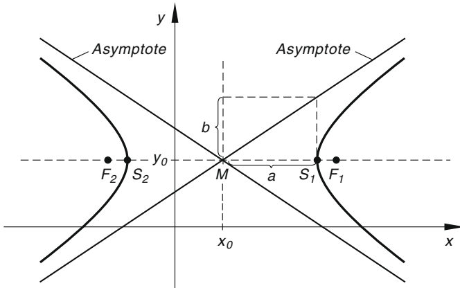
Bild III-97 Zur Hauptform der Hyperbelgleichung (verschobene Hyperbel)
