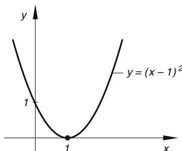
Bild III-8 Doppelte Nullstelle
