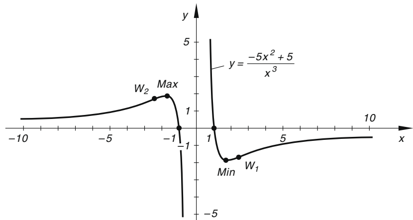
Bild IV-56 Funktionsgraph von y = \frac{-5x^2 + 5}{x^3} , x \neq 0
