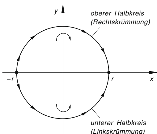
Bild IV-30 Zur Krümmung eines Kreises
