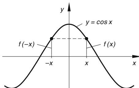
Bild III-11 Kosinusfunktion y = \cos x
