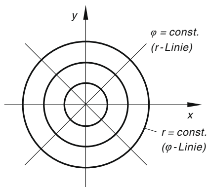
Bild III-38 Ebenes Polarkoordinatensystem
