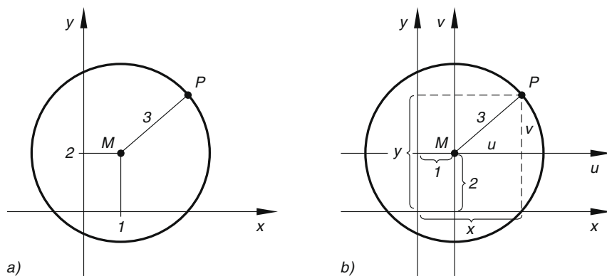
Bild III-32 Zur Koordinatentransformation eines Kreises
