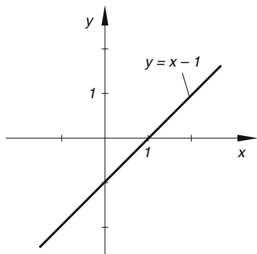
Bild III-51 Graph der „erweiterten“ Funktion y = x - 1
