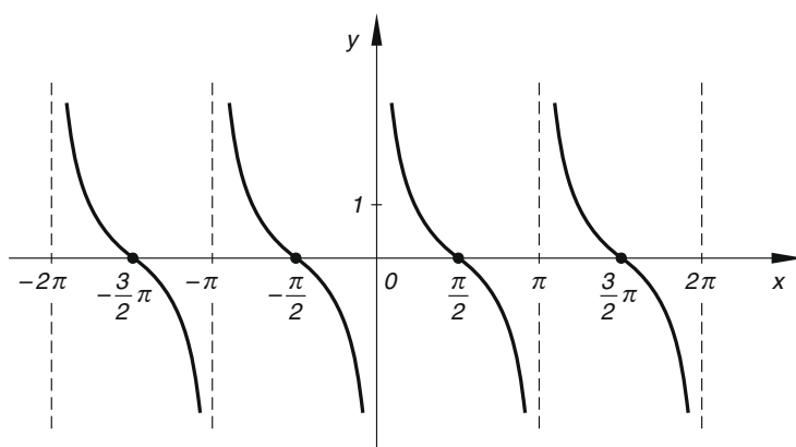
Bild III-114 Funktionsgraph der Kotangensfunktion
