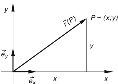
Bild II-22 Ortsvektor eines Punktes
