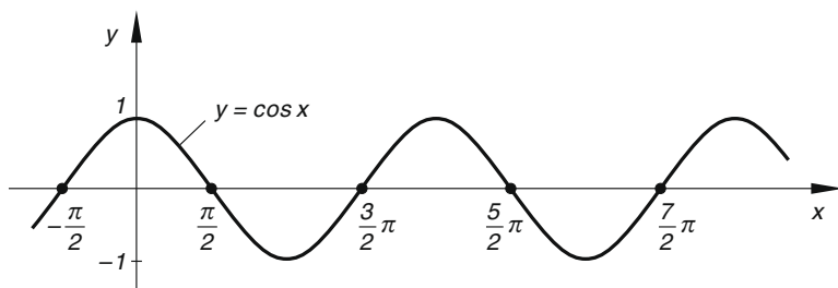
Bild III-147 Zur Lösung der Gleichung \cos x = 0
