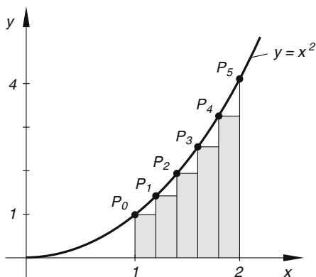
Bild V-4 Zum Begriff der Untersumme
