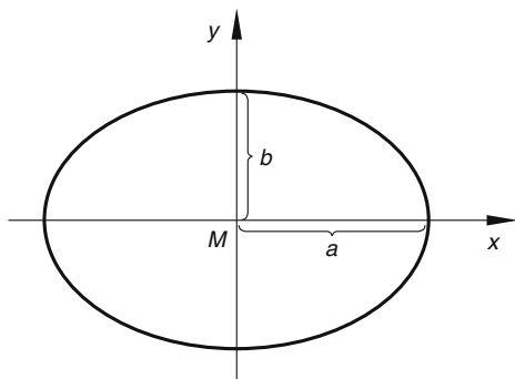
Bild III-93 Mittelpunktsellipse
