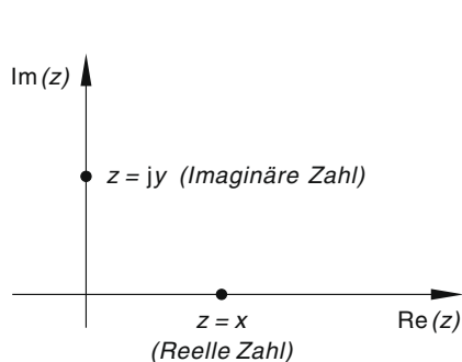
Bild VII-4 Bildliche Darstellung einer reellen bzw. imaginären Zahl
