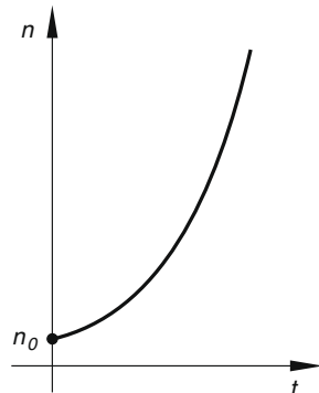
Bild III-159
