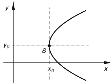
Bild III-100 Zur Hauptform der Parabelgleichung (verschobene Parabel)
