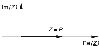
Bild VII-41 Ohmscher Widerstand
