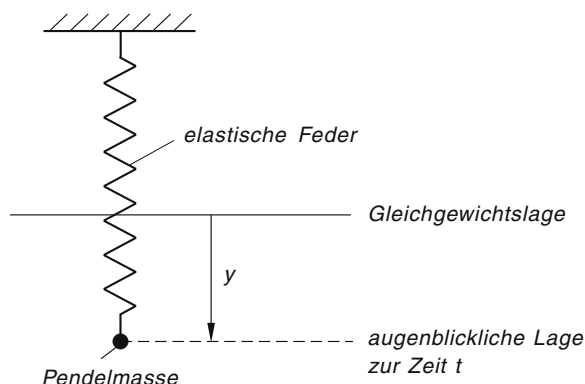
Bild III-124 Federpendel (Feder-Masse-Schwinger)
