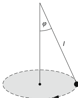
Bild VI-15 Konisches Pendel
