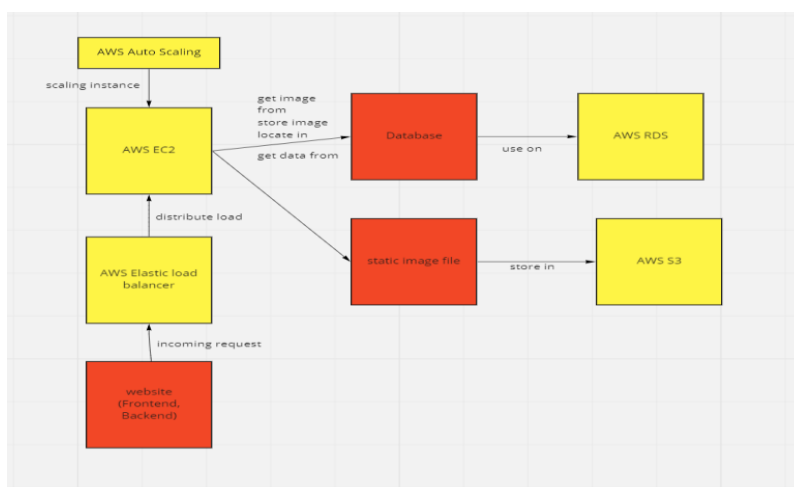
รูปที่ 3.7 โครงสร้างการใช้งาน AWS
