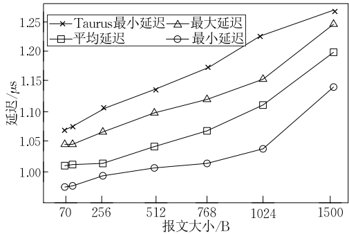
图 13 CAInNet 延迟性能评估
