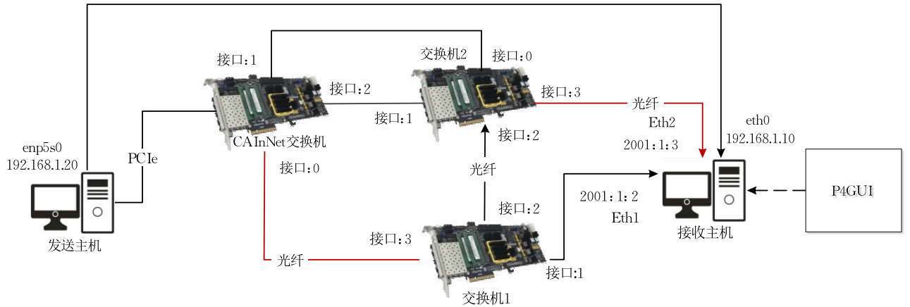
图 12 实验完整拓扑搭建
