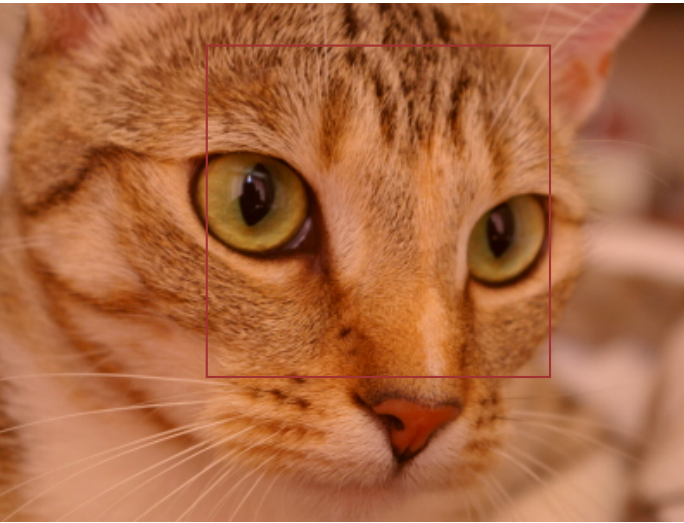
(d) Wavelet
