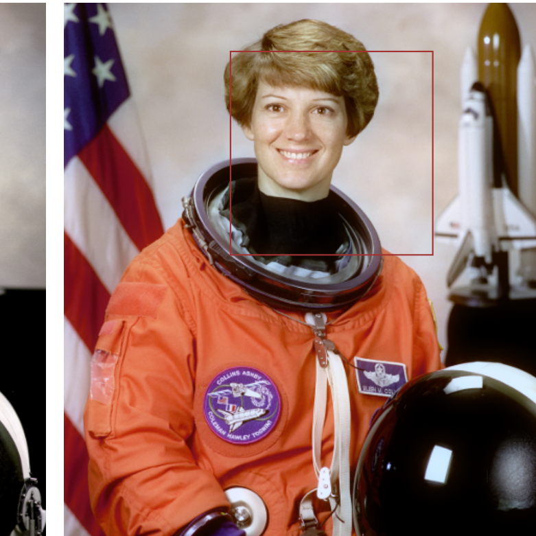
(d) Wavelet
