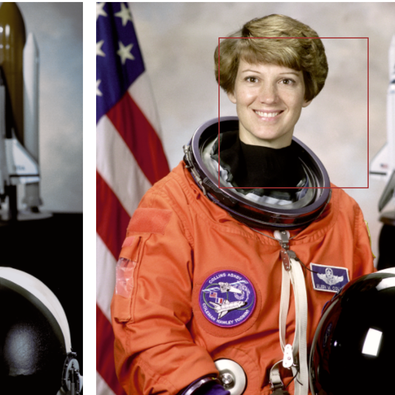
(h) ColorFM-O
