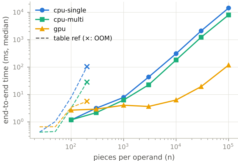
matmul_ii (ik,kj-&gt;ij)
