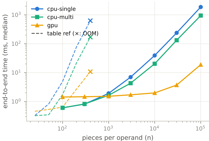
matvec_ii (ik,k-&gt;i)
