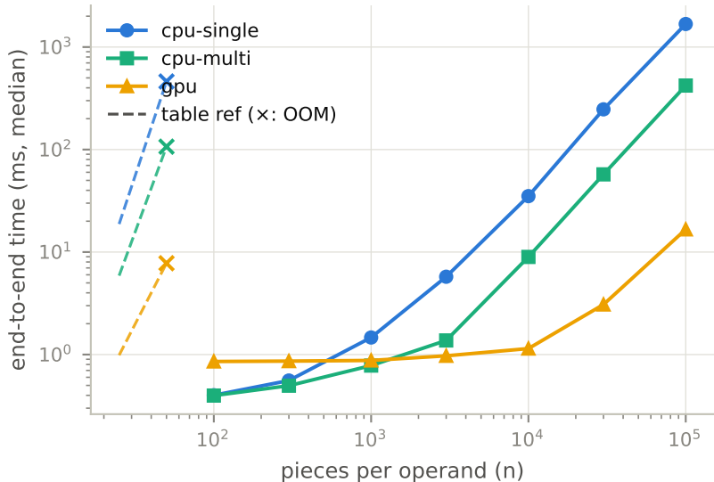
pointwise_2d_ii (ij,ij-&gt;ij)
