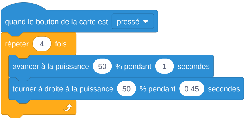
Programme du carré pour le mBot, en mode téléversé
