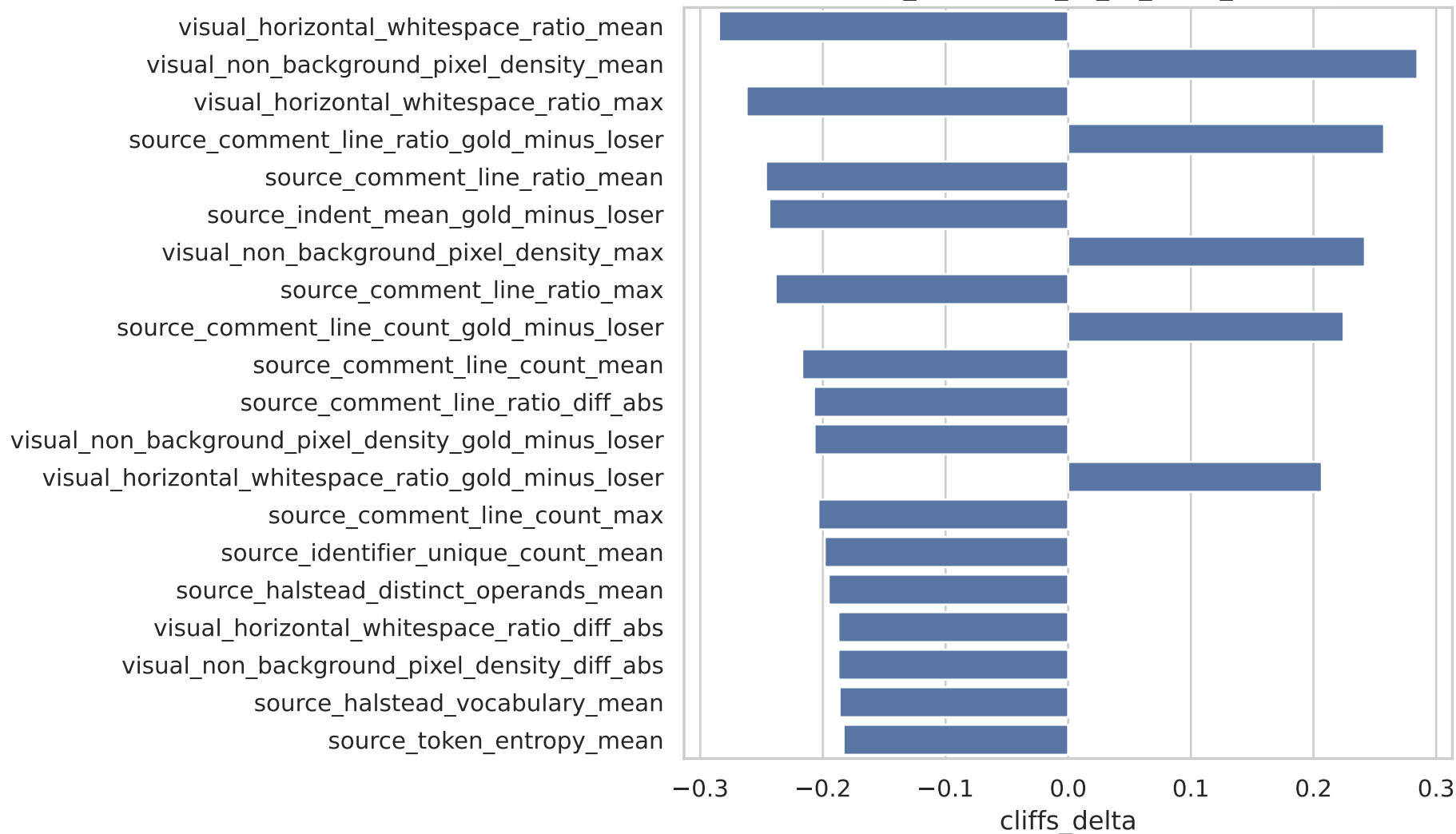
RFwrong_VLMrescue_vs_all_other_RFwrong
