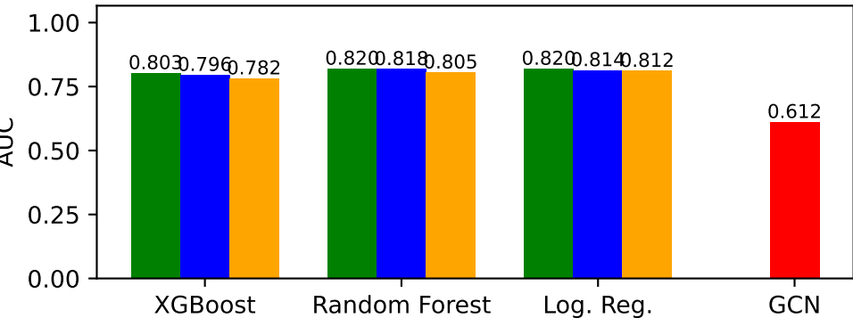
email-Eu — AUC
