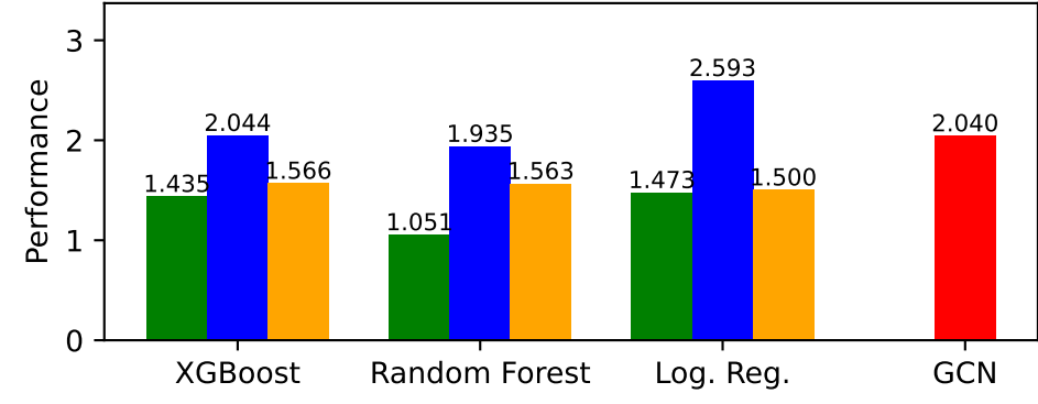
tags-ask-ubuntu — Performance
