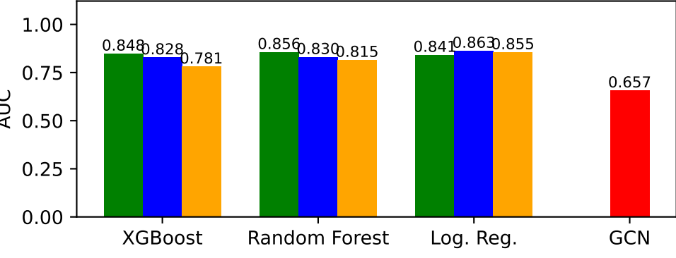
threads-ask-ubuntu — AUC
