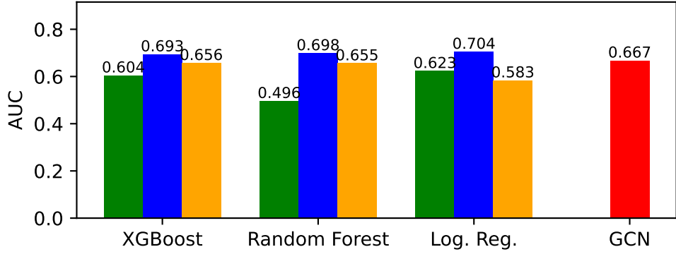
tags-ask-ubuntu — AUC
