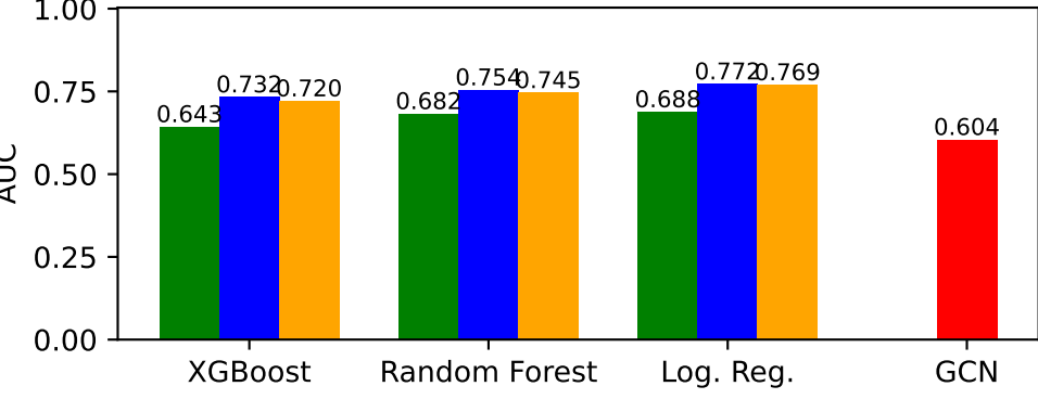
email-Enron — AUC
