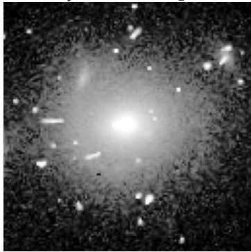
SLACS J1436-0000 \theta_E=1.12''
