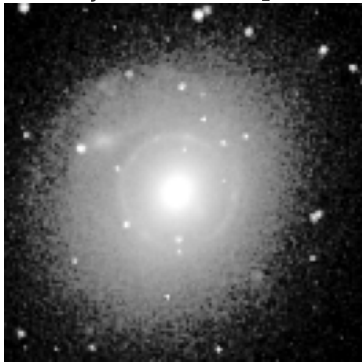
SLACS J1538+5817 \theta_E=1.00''
