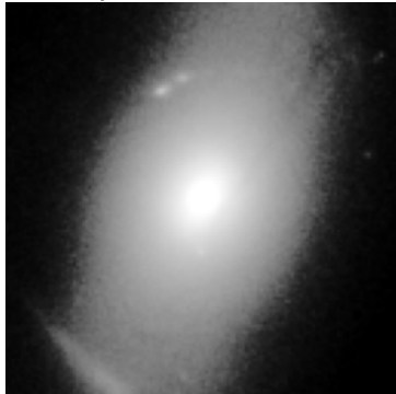
SLACS J0841+3824 \theta_E=1.41''
