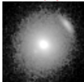
REAL Euclid Q1 \theta_E=1.67''
