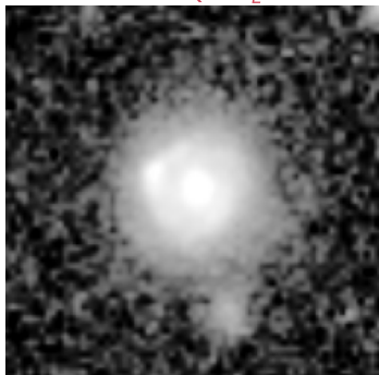
REAL Euclid Q1 \theta_E=0.63''
