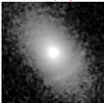
REAL Euclid Q1 \theta_E=1.21''
