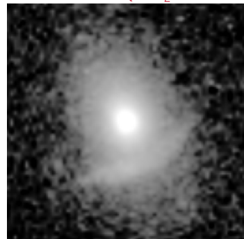
REAL Euclid Q1 \theta_E=0.94''
