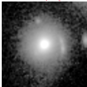
REAL Euclid Q1 \theta_E=1.31''
