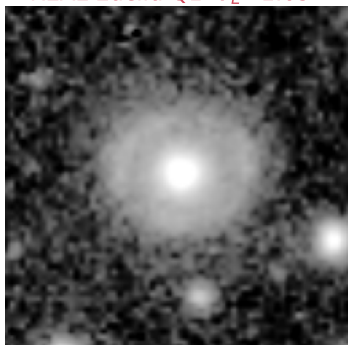
REAL Euclid Q1 \theta_E=1.09''
