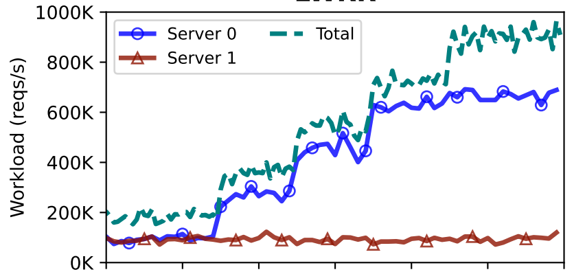
LWRR
