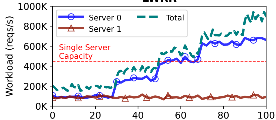
LWRR
