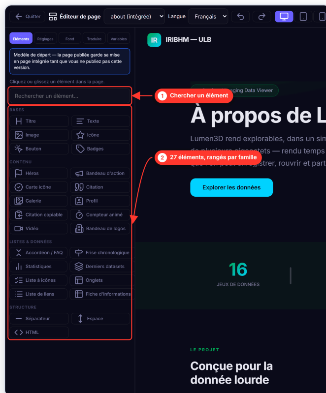
▲ La palette d'éléments.
