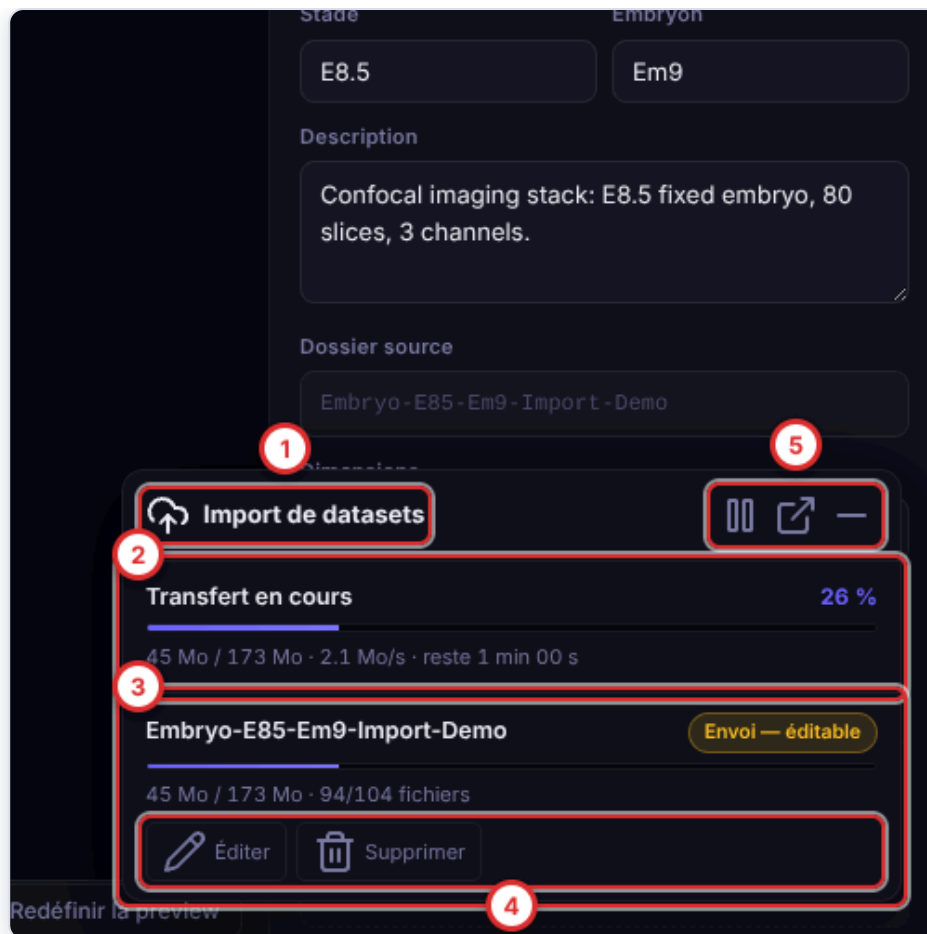
▲ Le panneau : une ligne par dataset, avec ses boutons.
