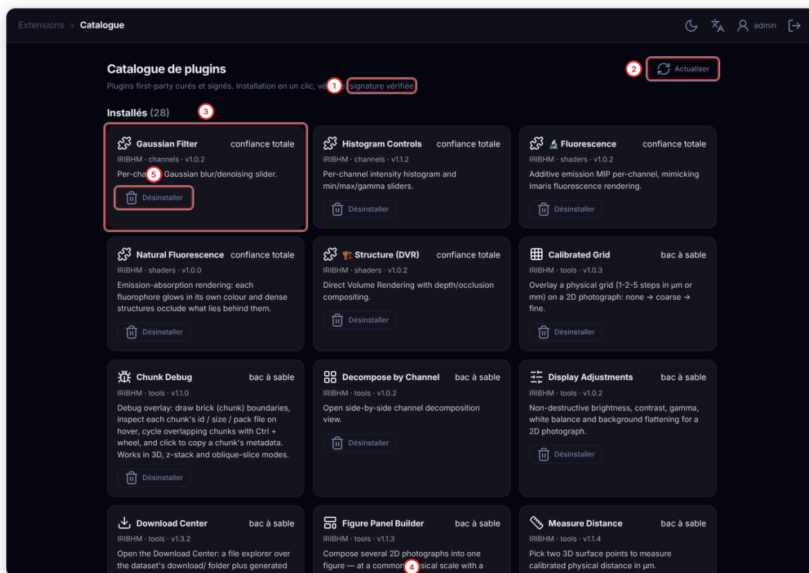
▲ L'onglet Catalogue (28 plugins installés).
