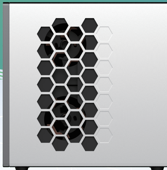
Model:MCAIPC1
