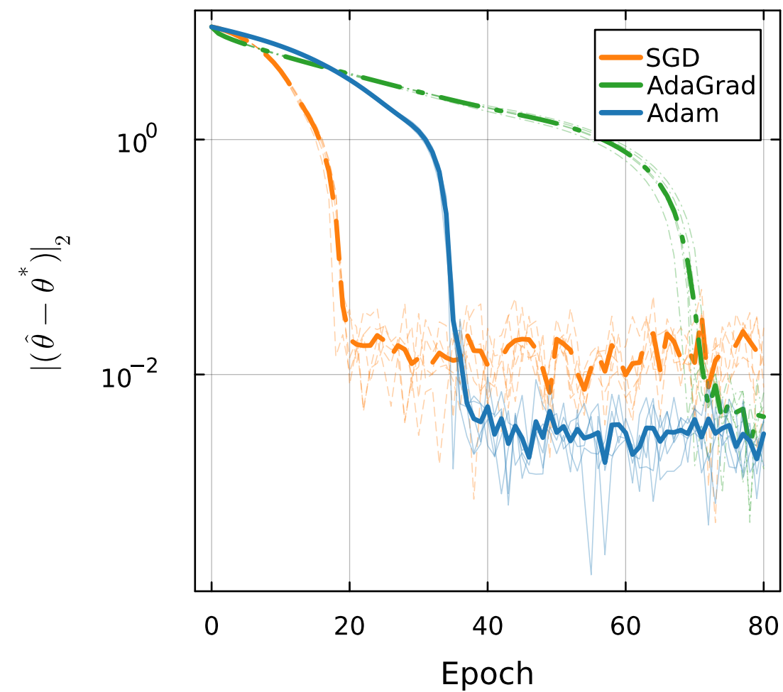
(b) Parameter error
