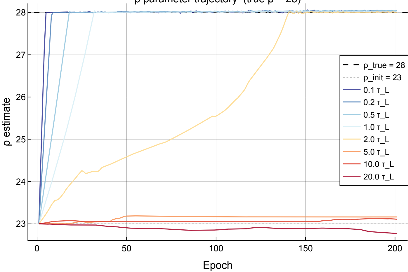
\rho parameter trajectory (true \rho = 28 )
