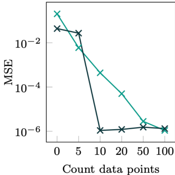
2D linear
