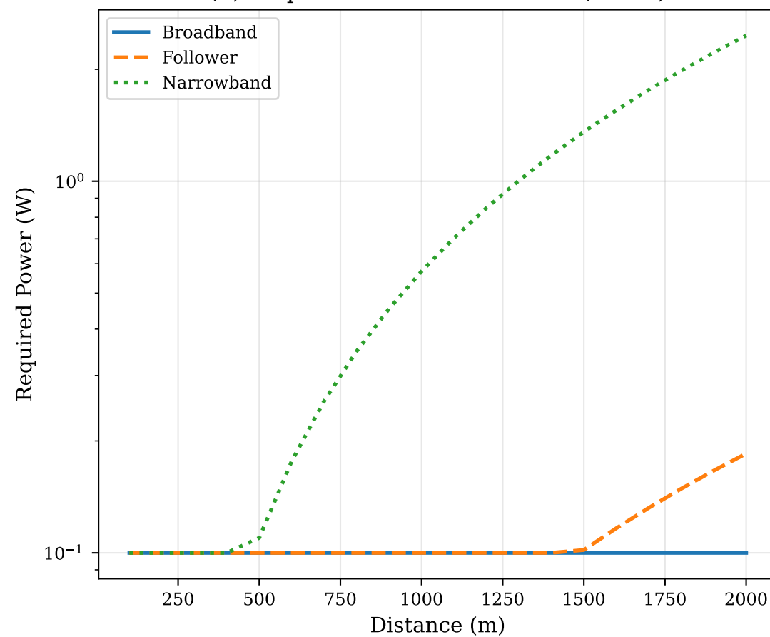
(d) Required Power vs Distance (FHSS)
