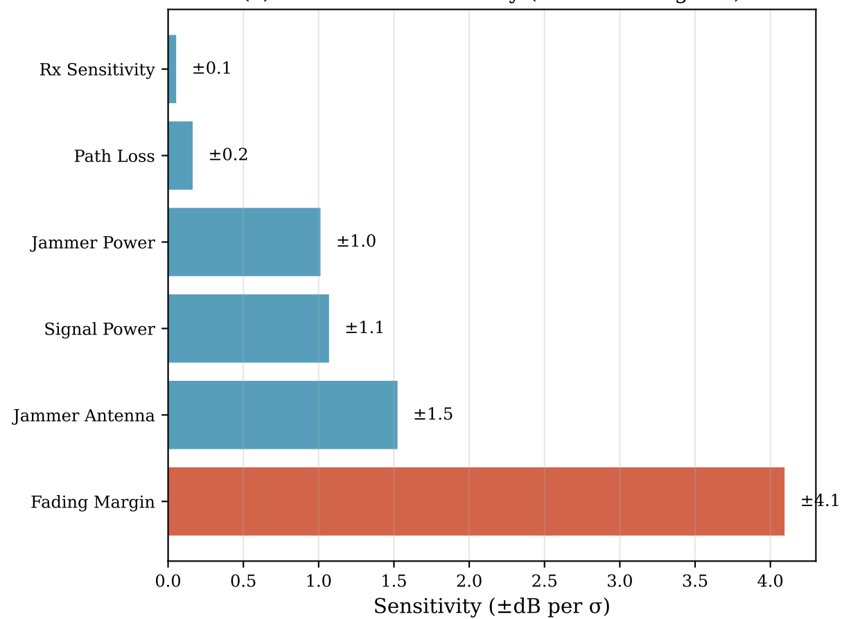
(c) Parameter Sensitivity (Tornado Diagram)
