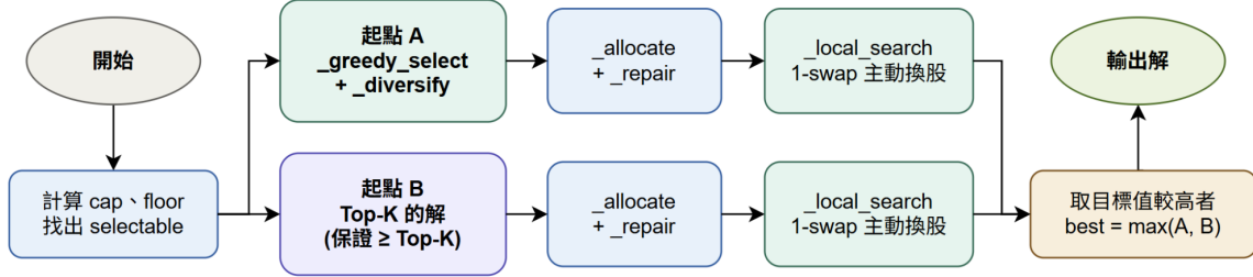
Figure 2: Greedy 多起點流程：起點 A 與起點 B 各經 ALLOCATE+REPAIR 與 1-swap LOCALSEARCH，最後取目標值較高者。
