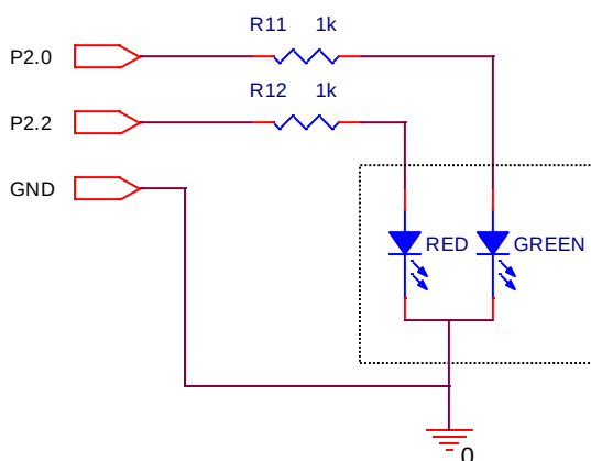
Fig. 3.2.1.b. Output module
