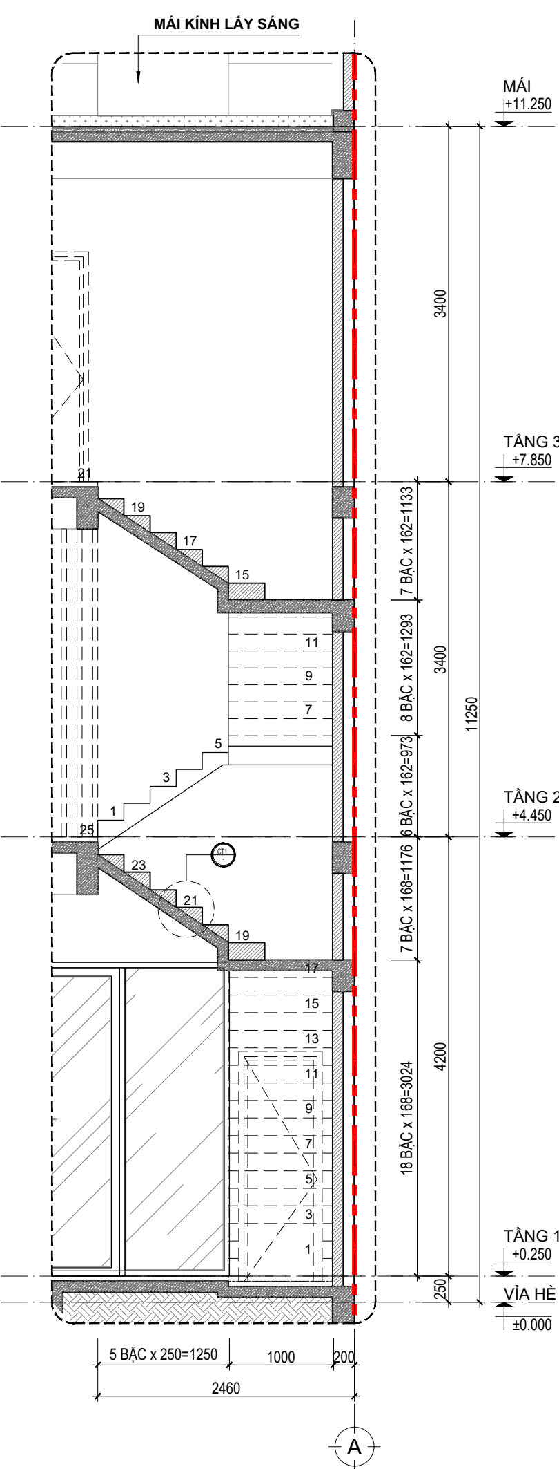
MẶT CẮT 2-2_TL:1/50
