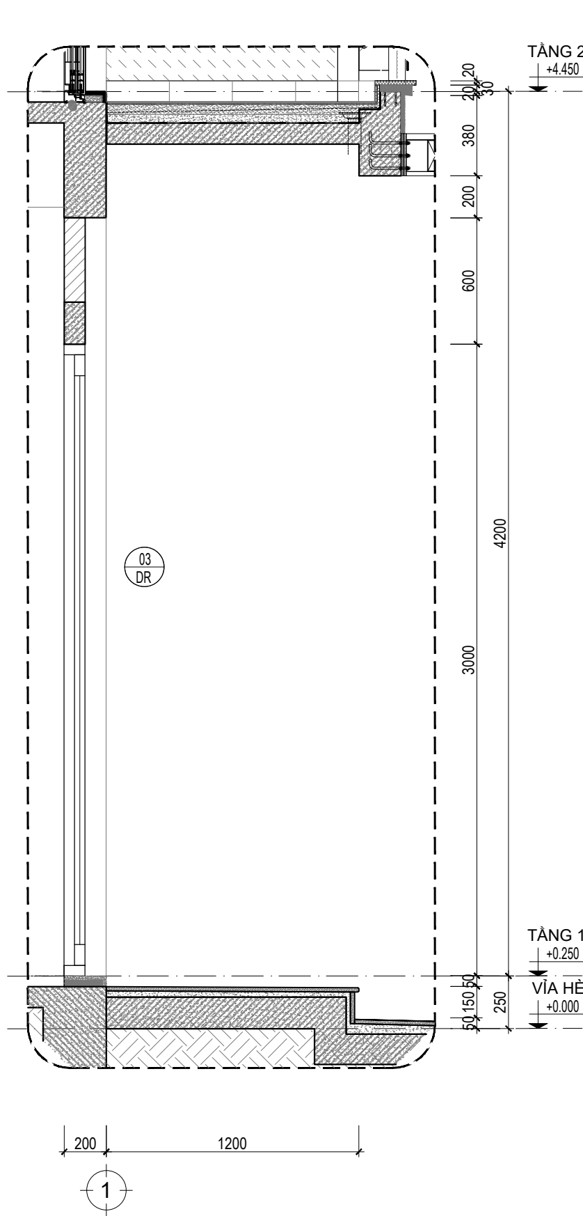
M. CẮT TRÍCH ĐOẠN 1-1_TL:1/25
