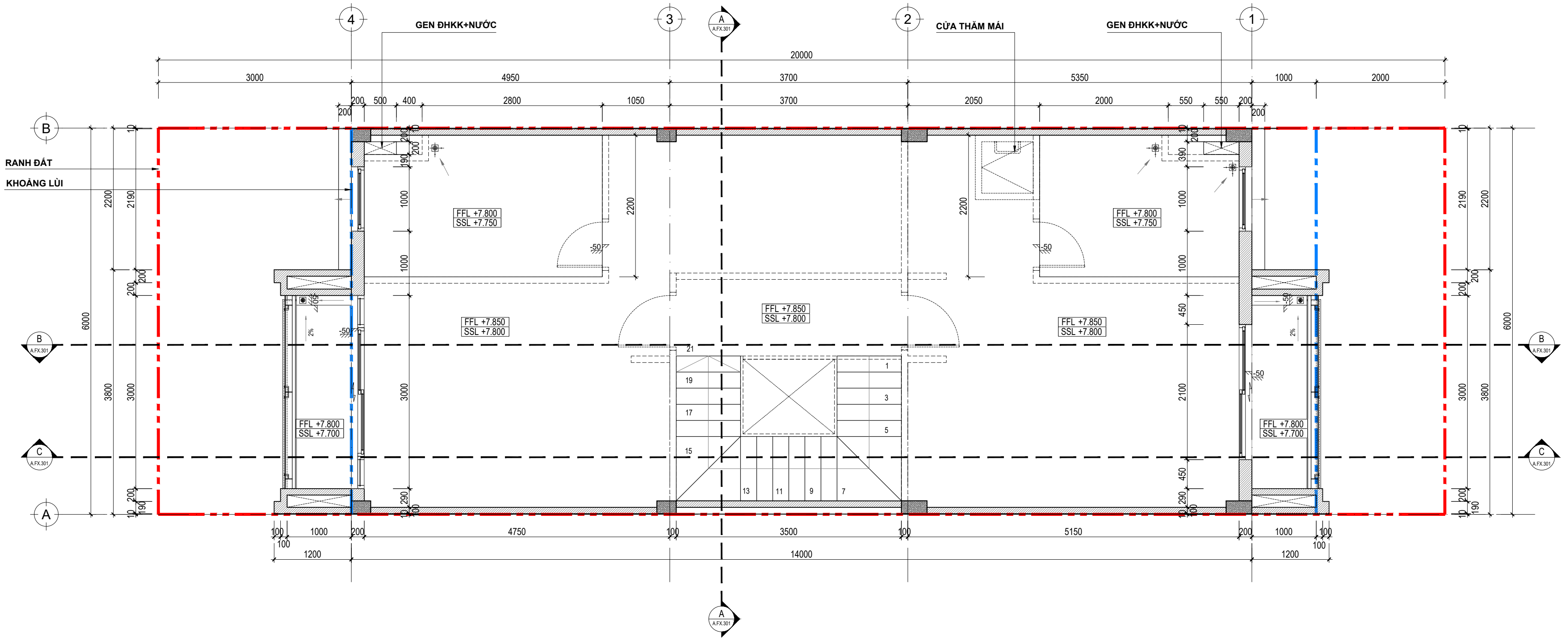
MẶT BẰNG KÍCH THƯỚC TẦNG 3 _ TL:1/50
