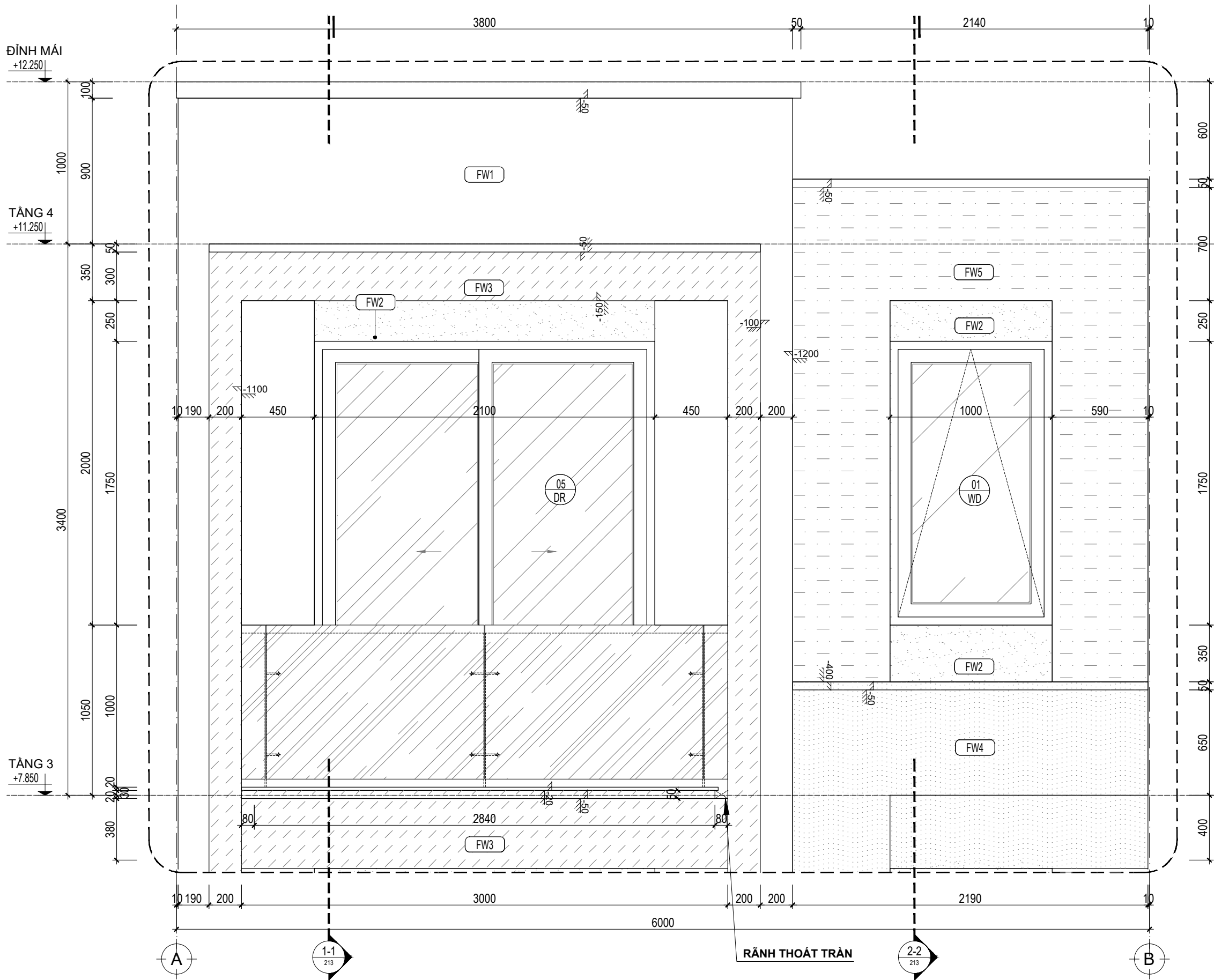
MẶT ĐỨNG TRÍCH ĐOẠN A-B - TẦNG 3_TL:1/25
