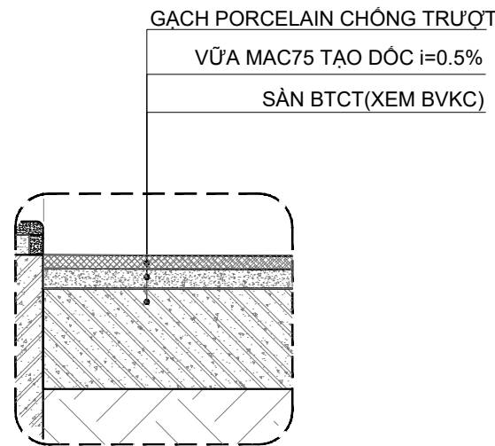
CHI TIẾT 1_TL:1/10
