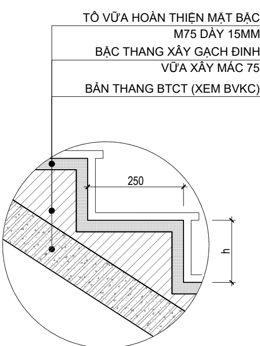
CHI TIẾT 1_TL:1/10
