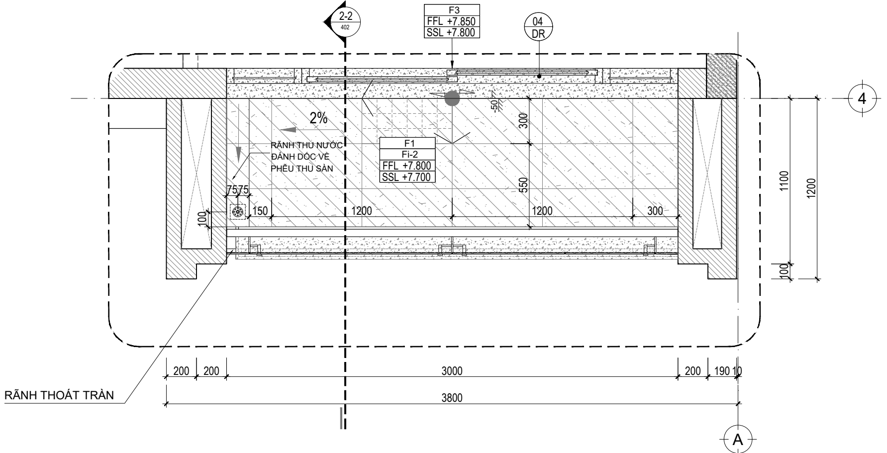
MẶT BẰNG BAN CÔNG TẦNG 3 ĐIỂN HÌNH_TL:1/25
