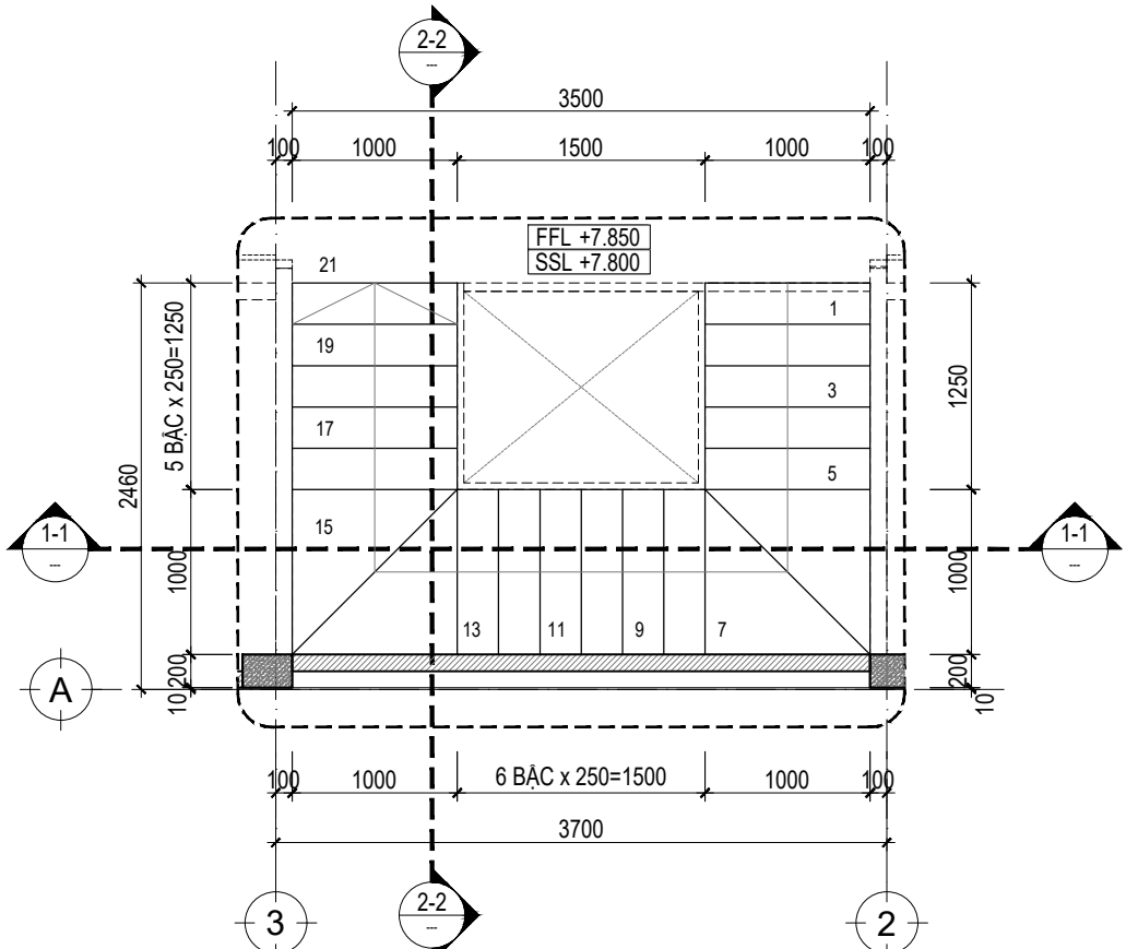
MẶT BẰNG THANG TẦNG 3_TL:1/50
