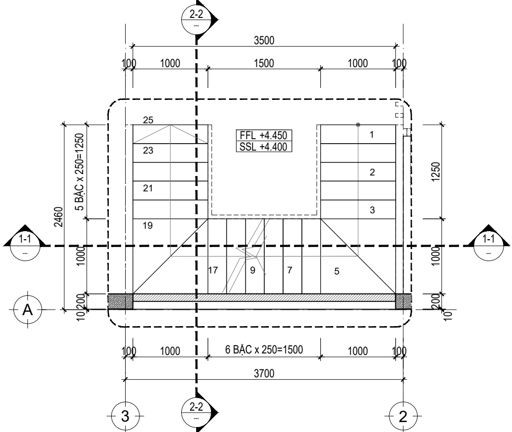
MẶT BẰNG THANG TẦNG 2_TL:1/50
