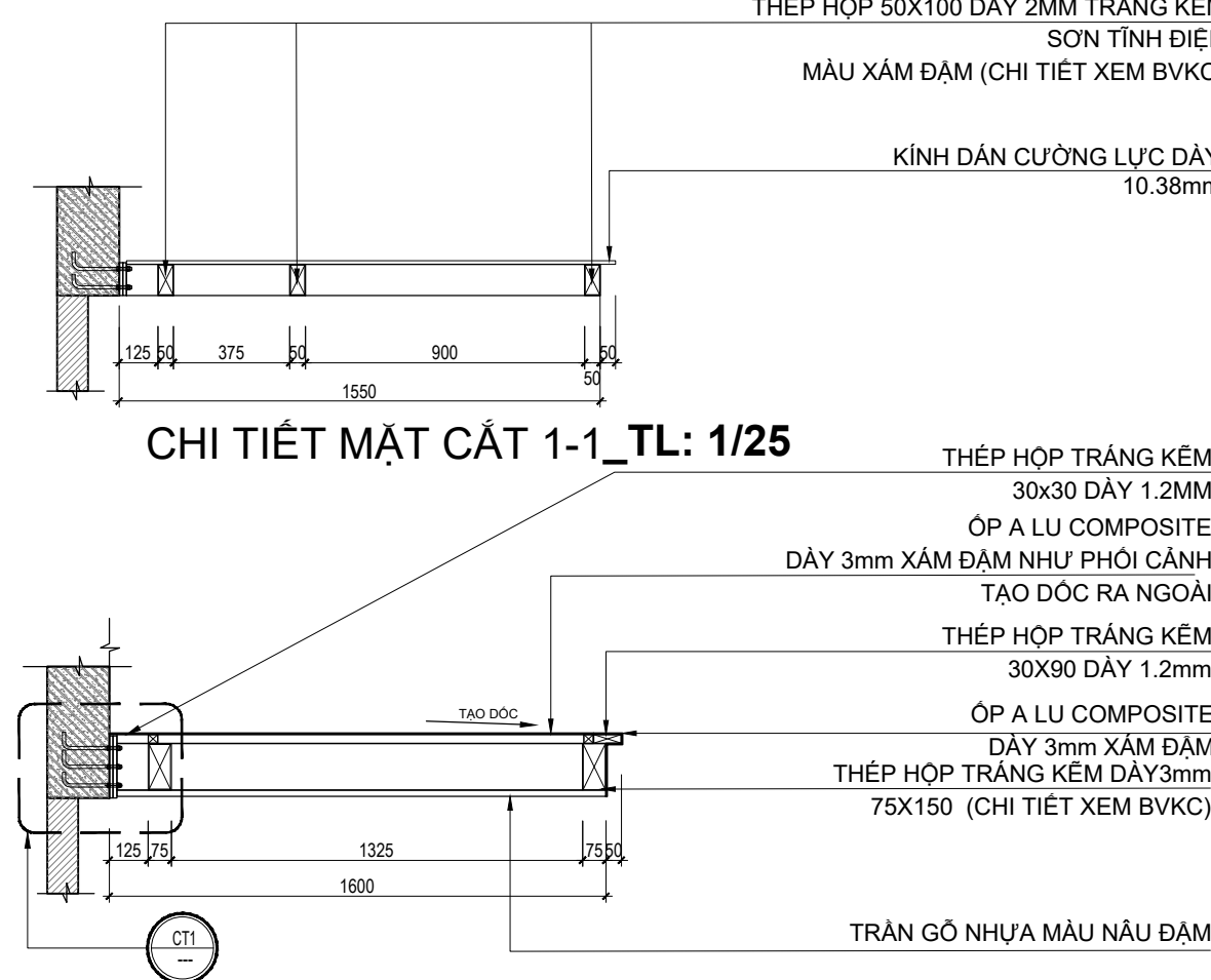
CHI TIẾT MẶT CẮT 2-2_TL: 1/25
