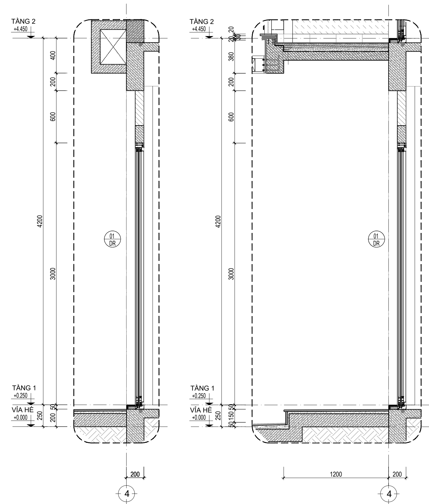
M. CẮT TRÍCH ĐOẠN 2-2_TL:1/25
