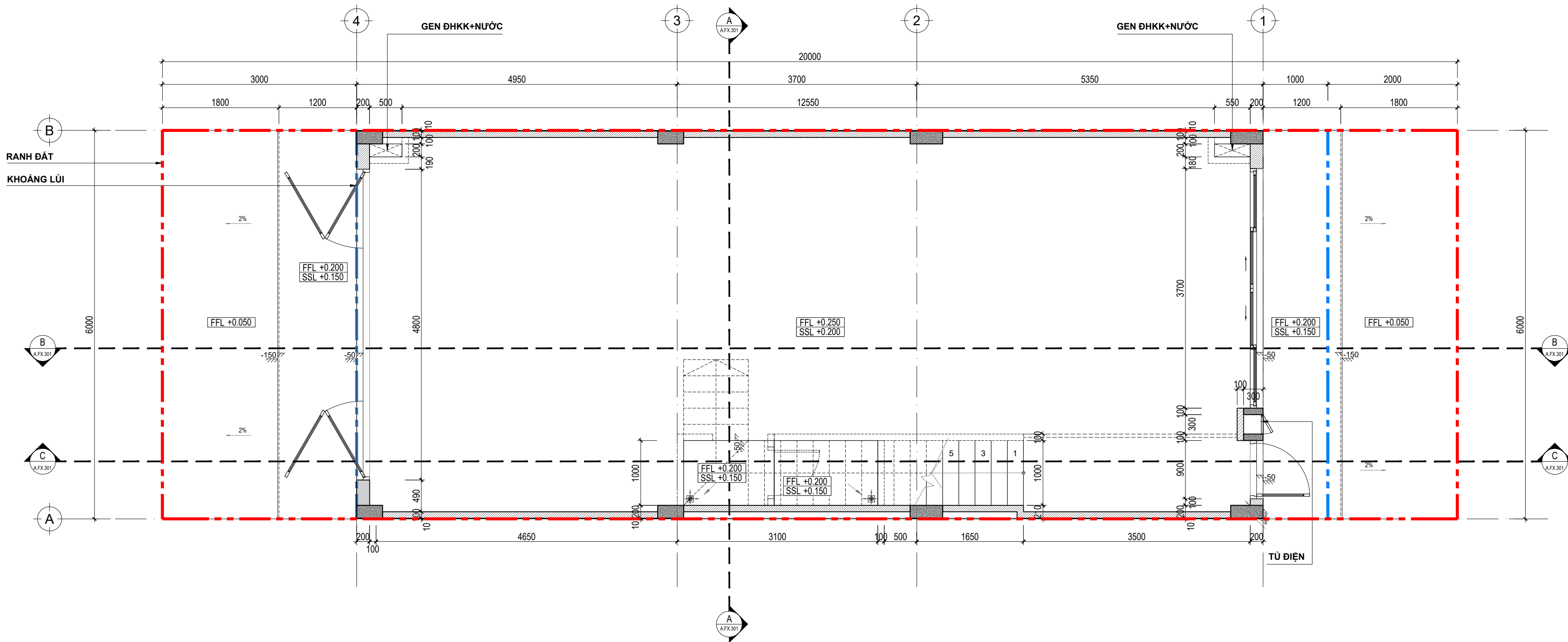
MẶT BẰNG KÍCH THƯỚC TẦNG 1 _ TL:1/50
