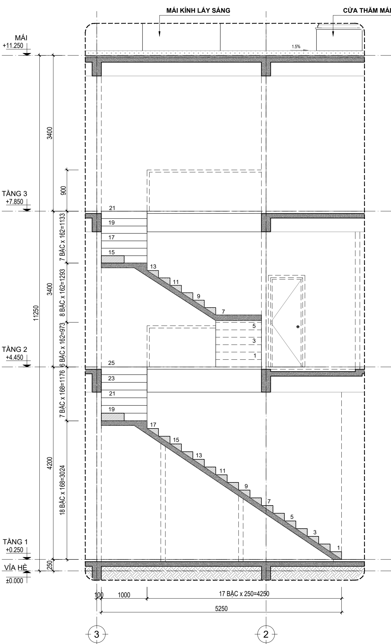
MẶT CẮT 1-1_TL:1/50
