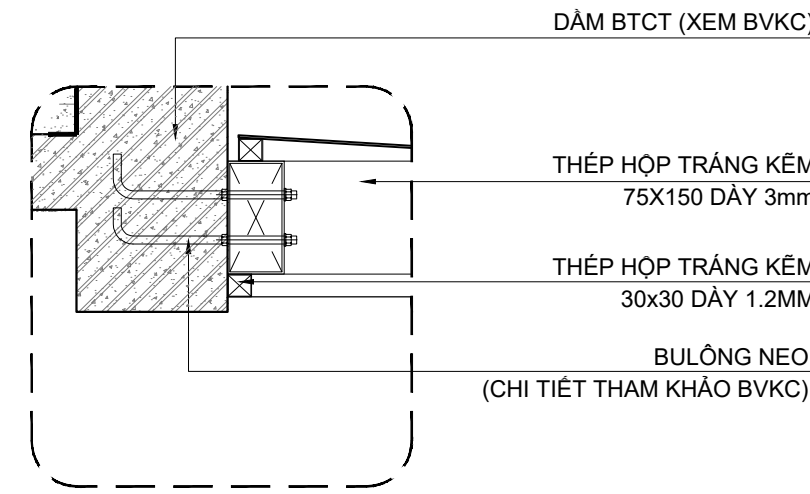
CHI TIẾT 1_TL: 1/10
