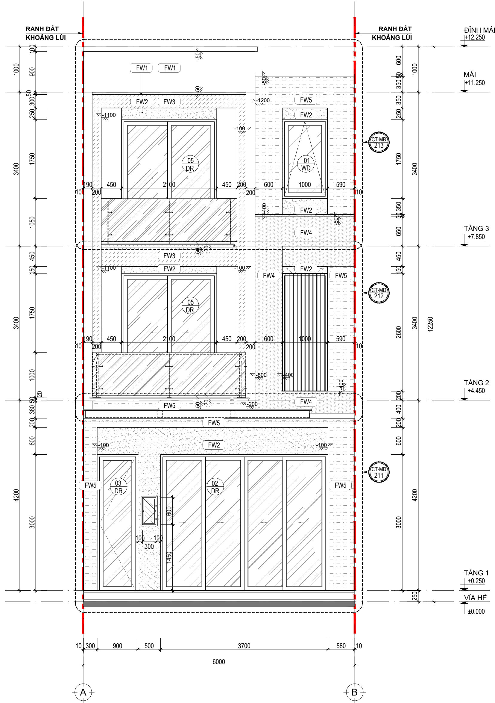
MẶT ĐƯNG A-B _ TL:1/50
