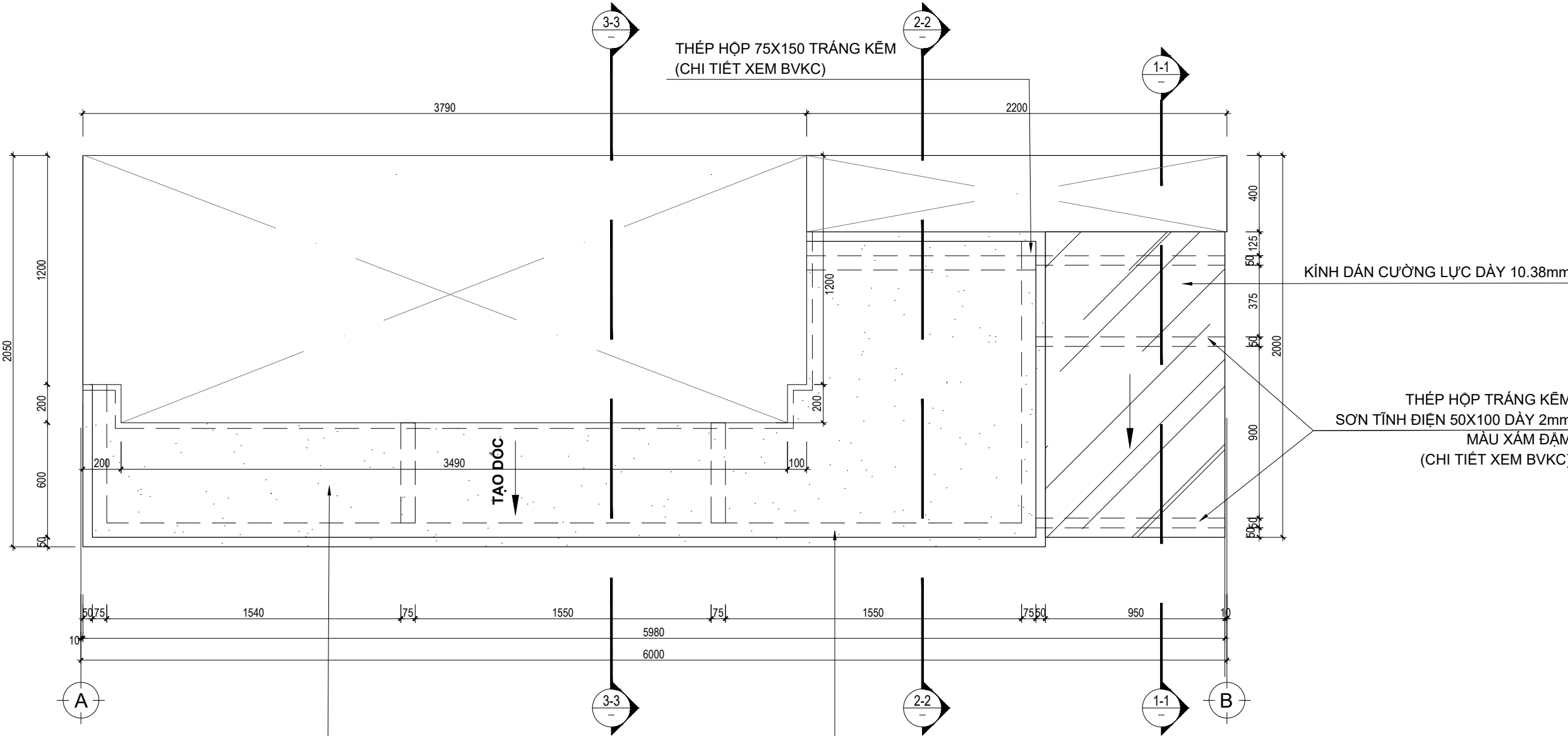
CHI TIẾT MẶT BẰNG MÁI ĐÓN TRỰC A-B_TL: 1/25
