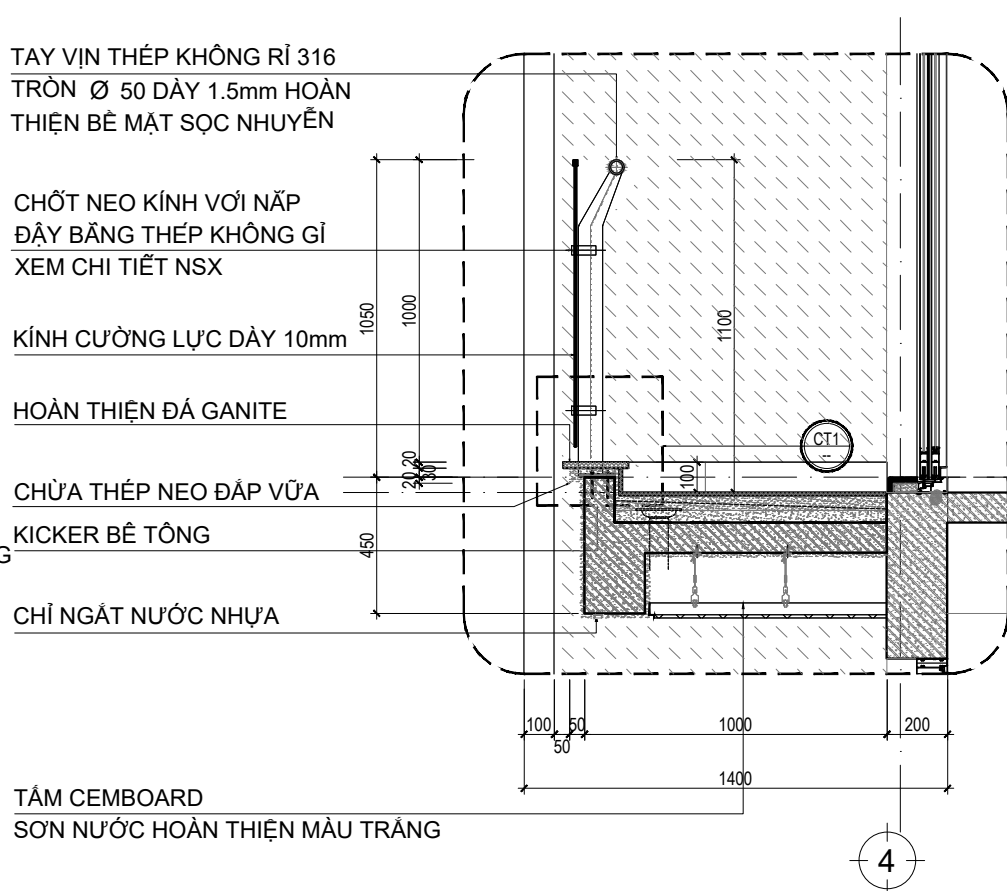
MC 2-2 BAN CÔNG TẦNG 3_TL:1/25
