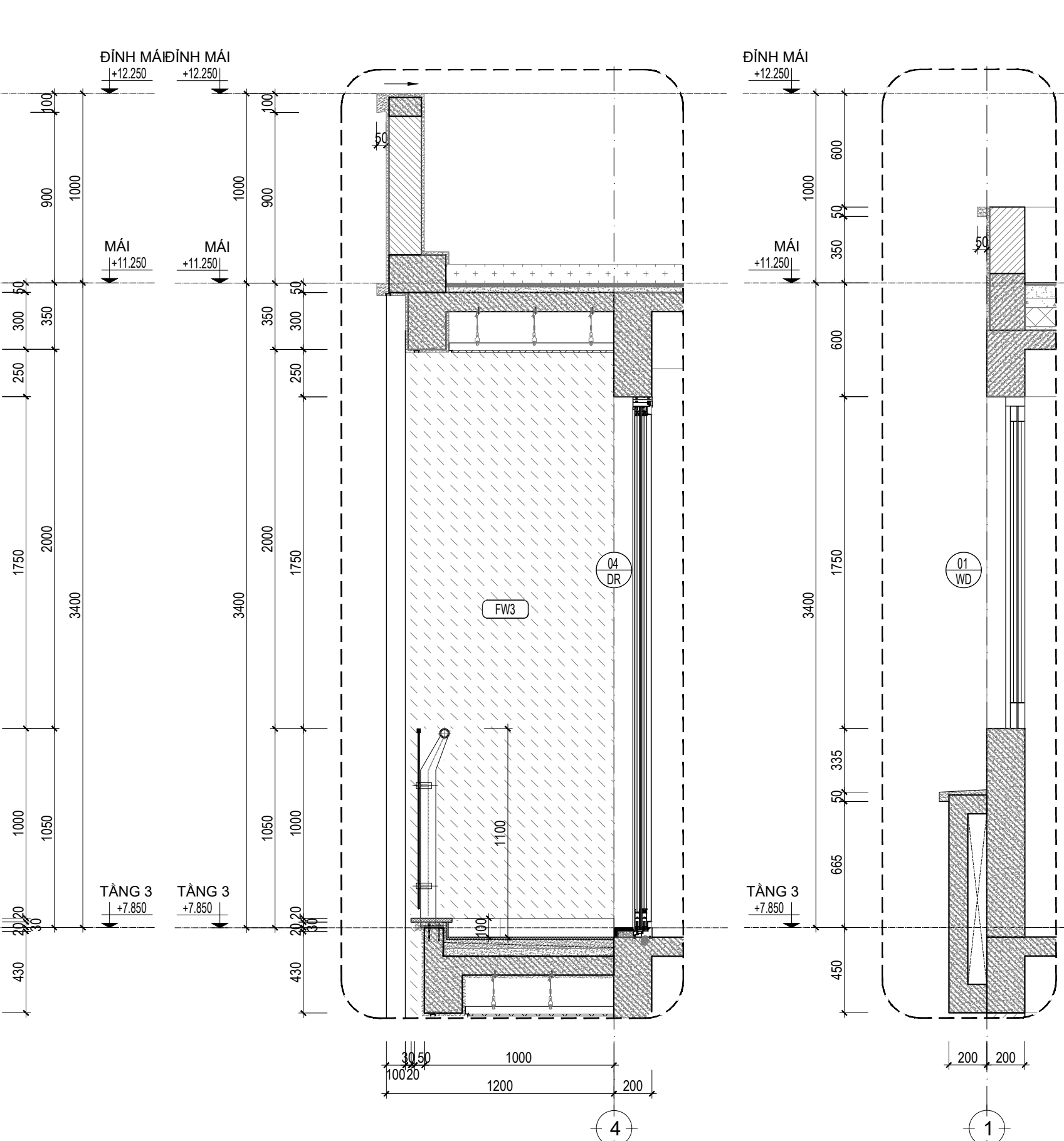
M. CẮT TRÍCH ĐOẠN 1-1_TL:1/25 M. CẮT TRÍCH ĐOẠN 2-2_TL:1/25
