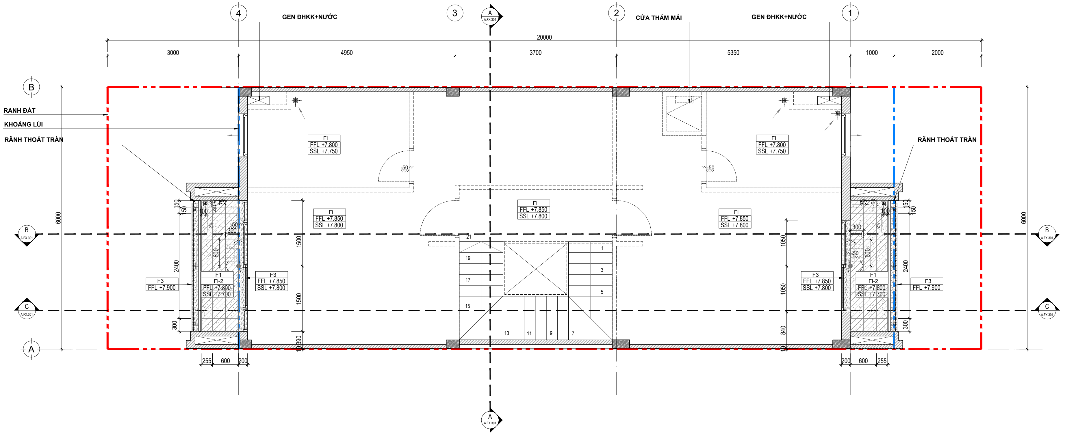
MẶT BẰNG HOÀN THIỆN SÀN TẦNG 3 _ TL:1/50
