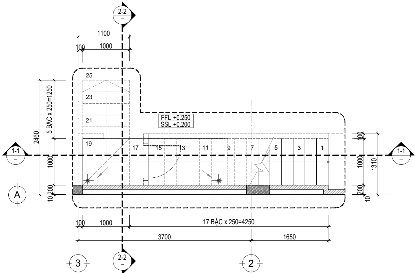
MẶT BẰNG THANG TẦNG 1_TL:1/50
