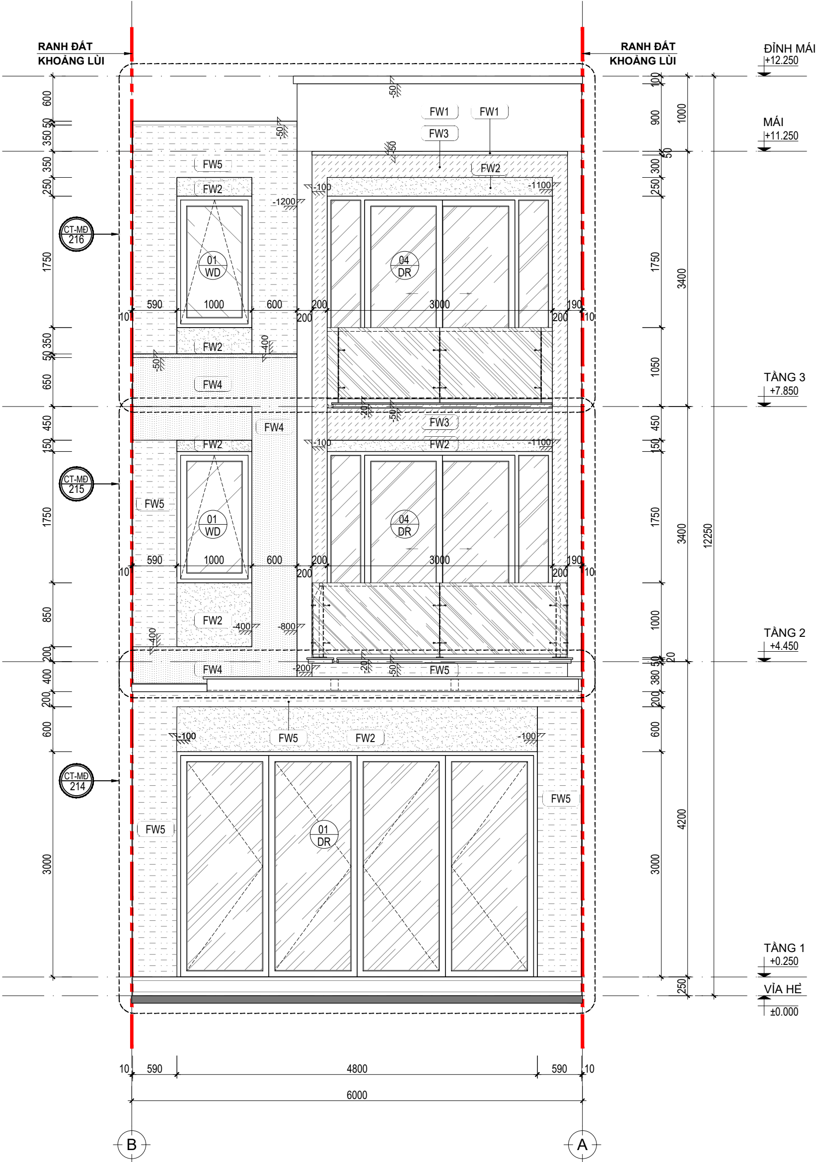
MẶT ĐỨNG B-A _ TL:1/50
