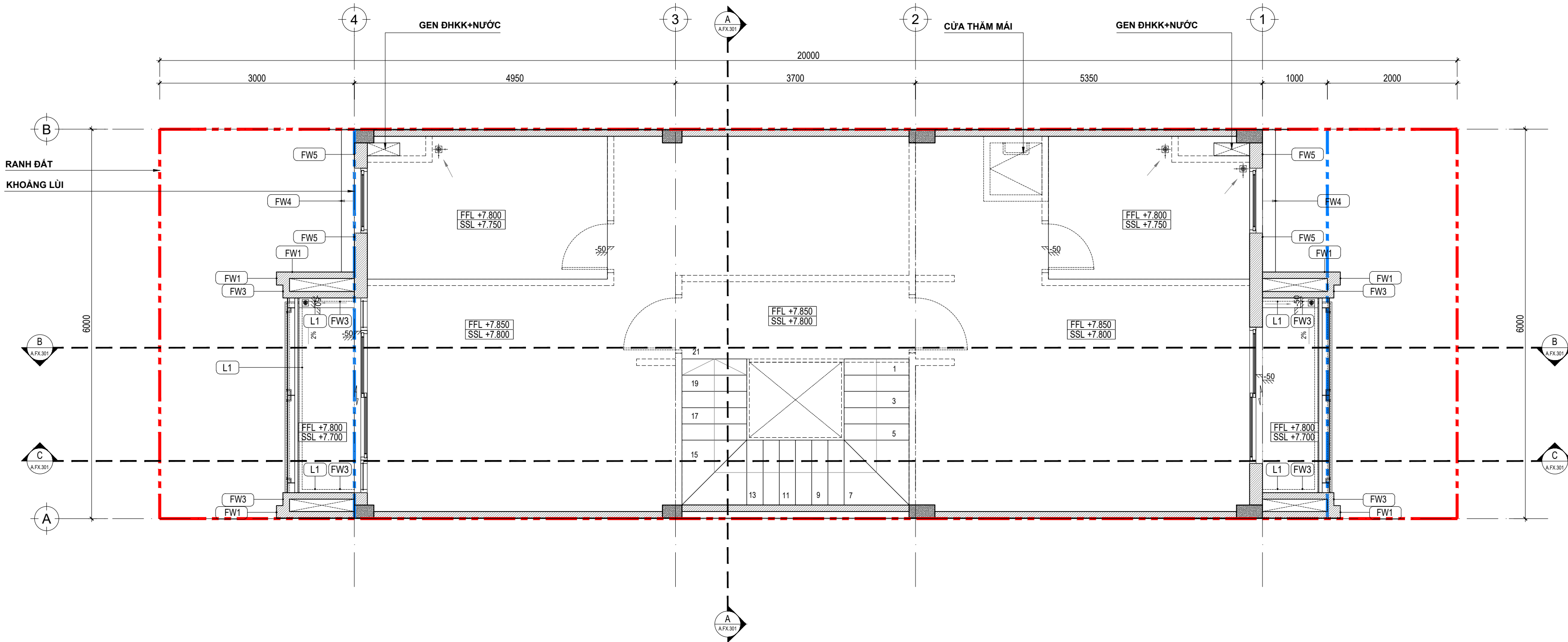
MẶT BẰNG HOÀN THIỆN TƯỜNG TẦNG 3 _ TL:1/50
