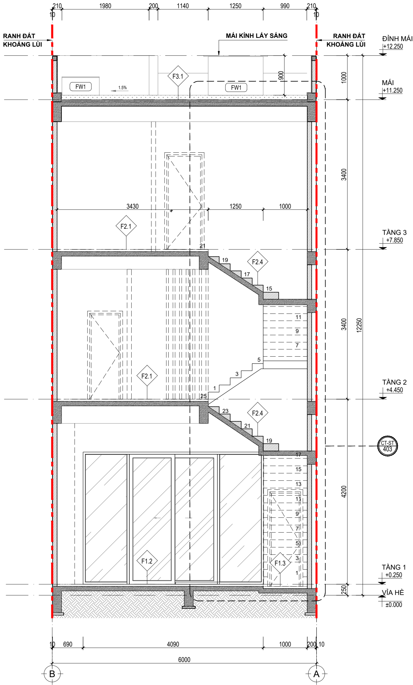
MẶT CẮT A-A _ TL:1/50
