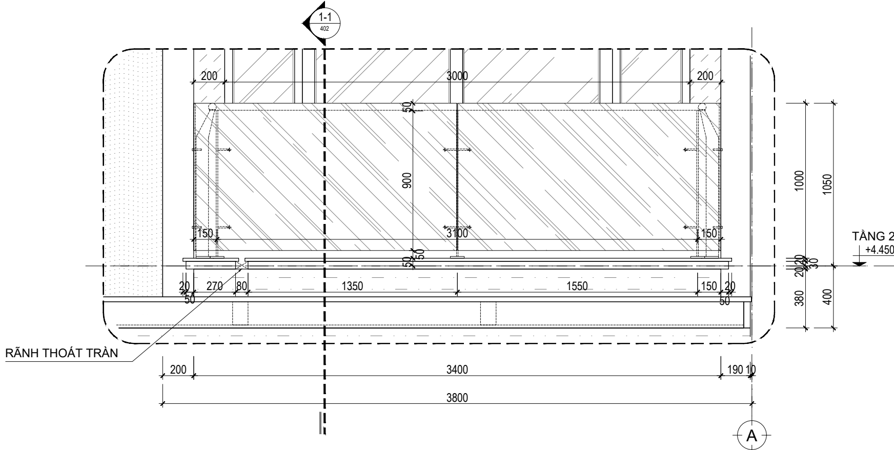
MẶT ĐỨNG BAN CÔNG TẦNG 2 ĐIỂN HÌNH_TL:1/25
