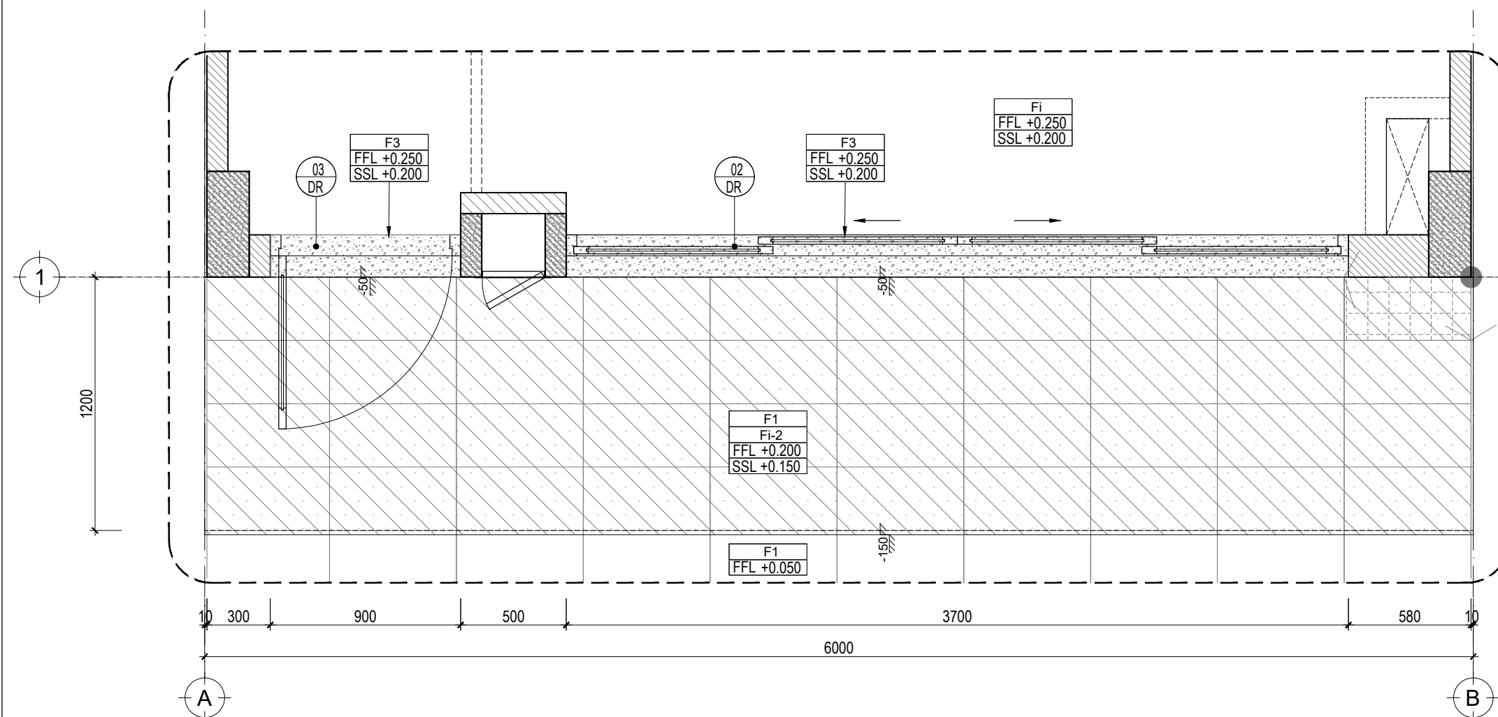
MẶT BẰNG TRÍCH ĐOẠN A-B- TẦNG 1_TL:1/25
