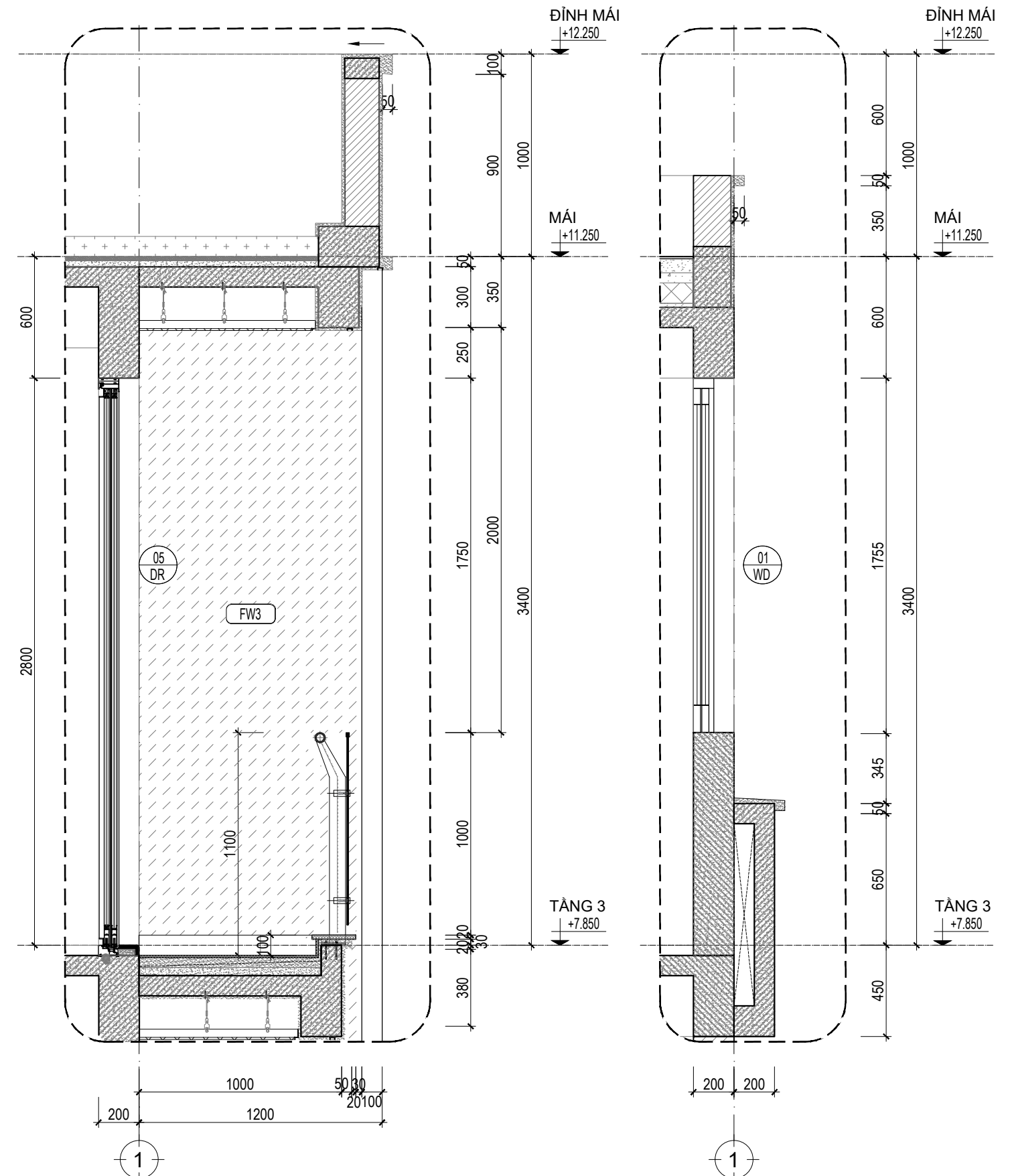
M. CẮT TRÍCH ĐOẠN 1-1_TL:1/25
