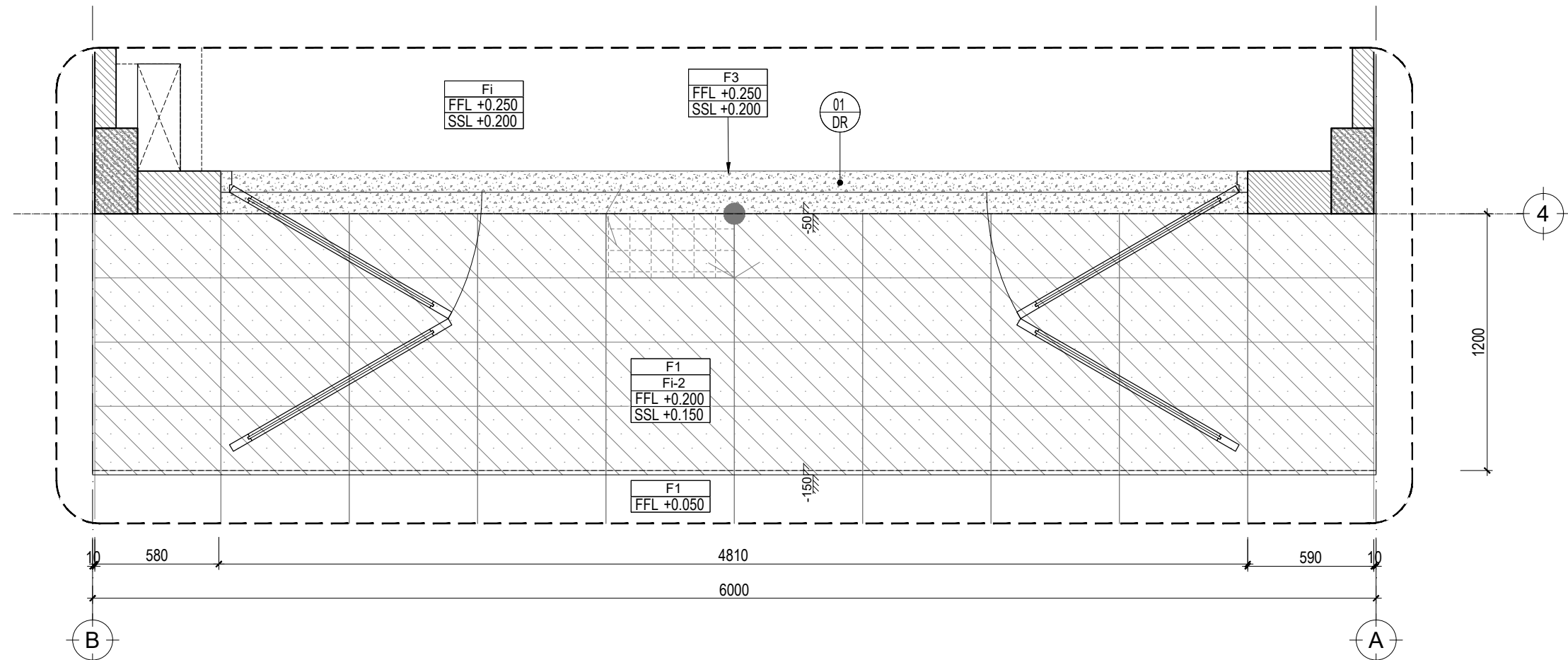
MẶT BẰNG TRÍCH ĐOẠN B-A - TẦNG 1_TL:1/25
