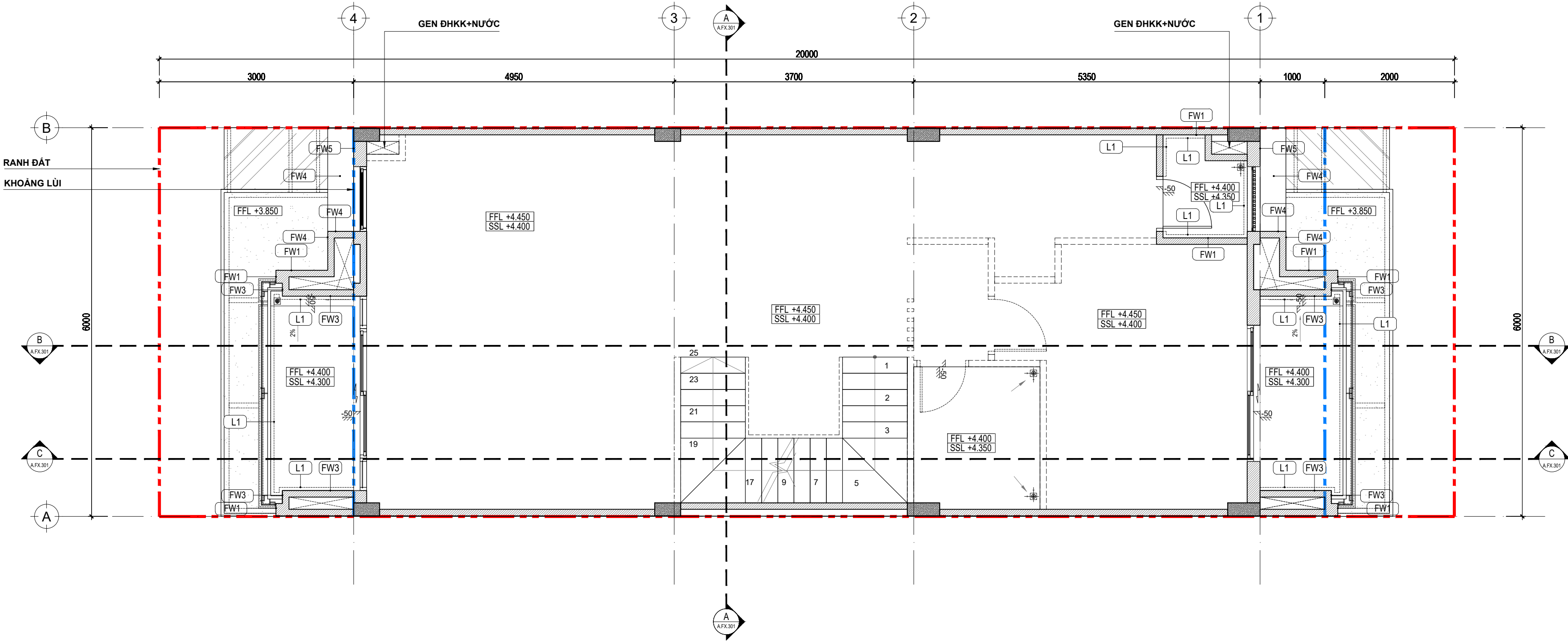
MẶT BẰNG HOÀN THIỆN TƯỜNG TẦNG 2 _ TL:1/50
