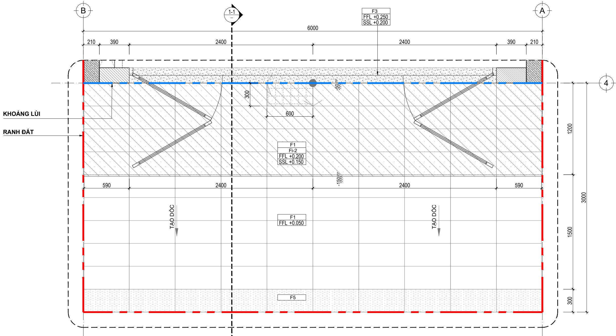
MẶT BẰNG SÂN TRƯỚC_TL:1/25
