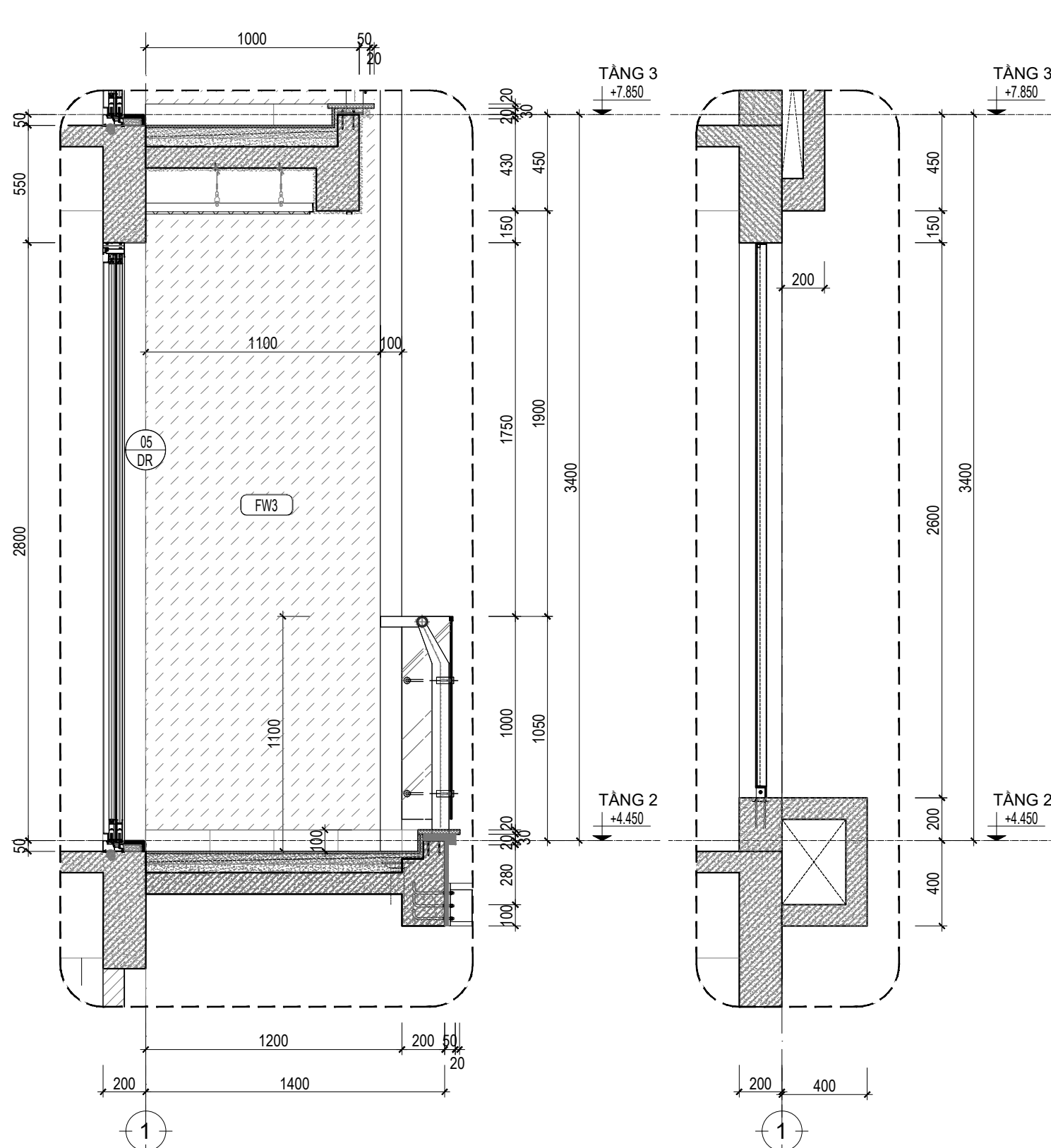
M. CẮT TRÍCH ĐOẠN 1-1_TL:1/25
