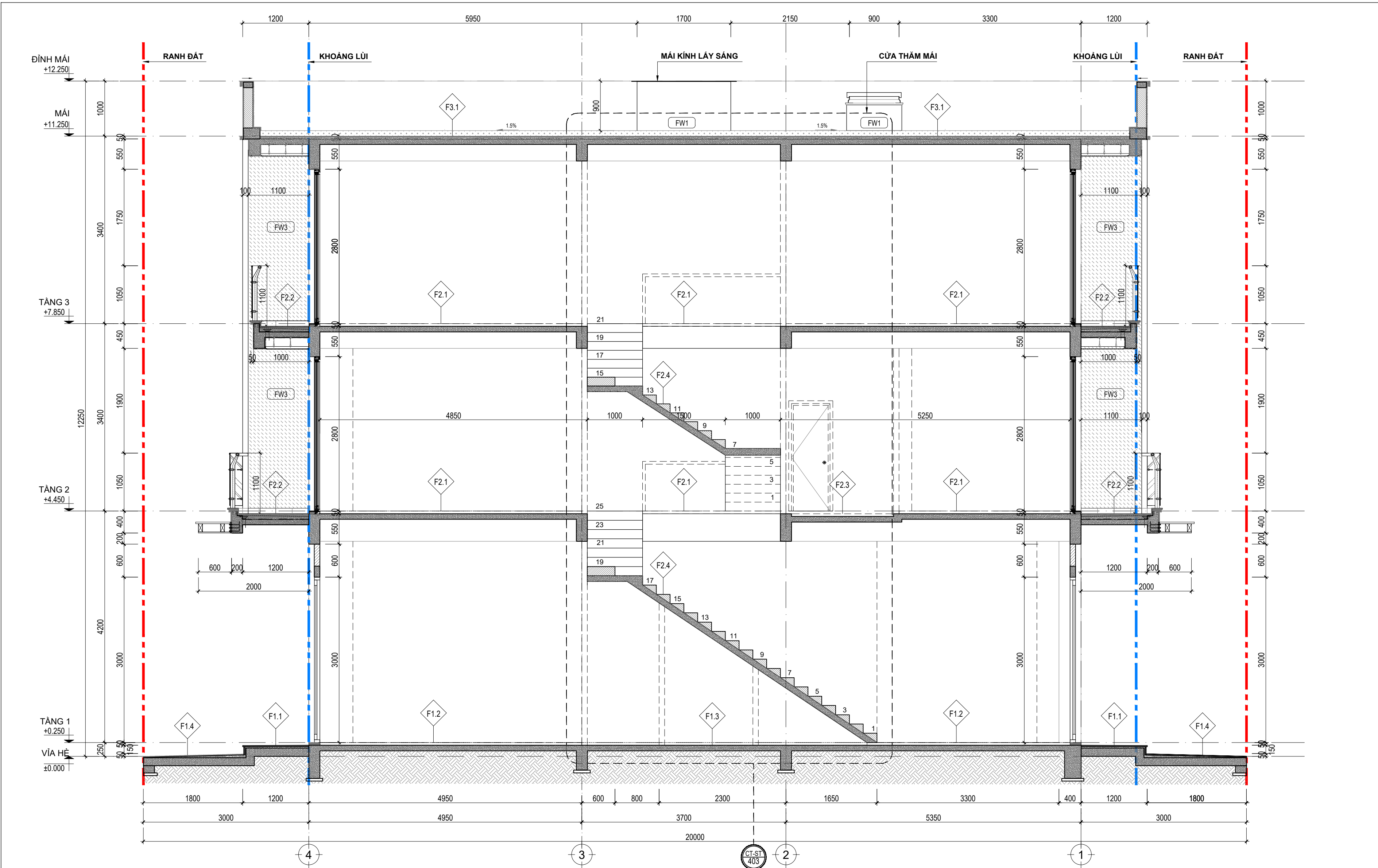
MẶT CẮT C-C _ TL:1/50
