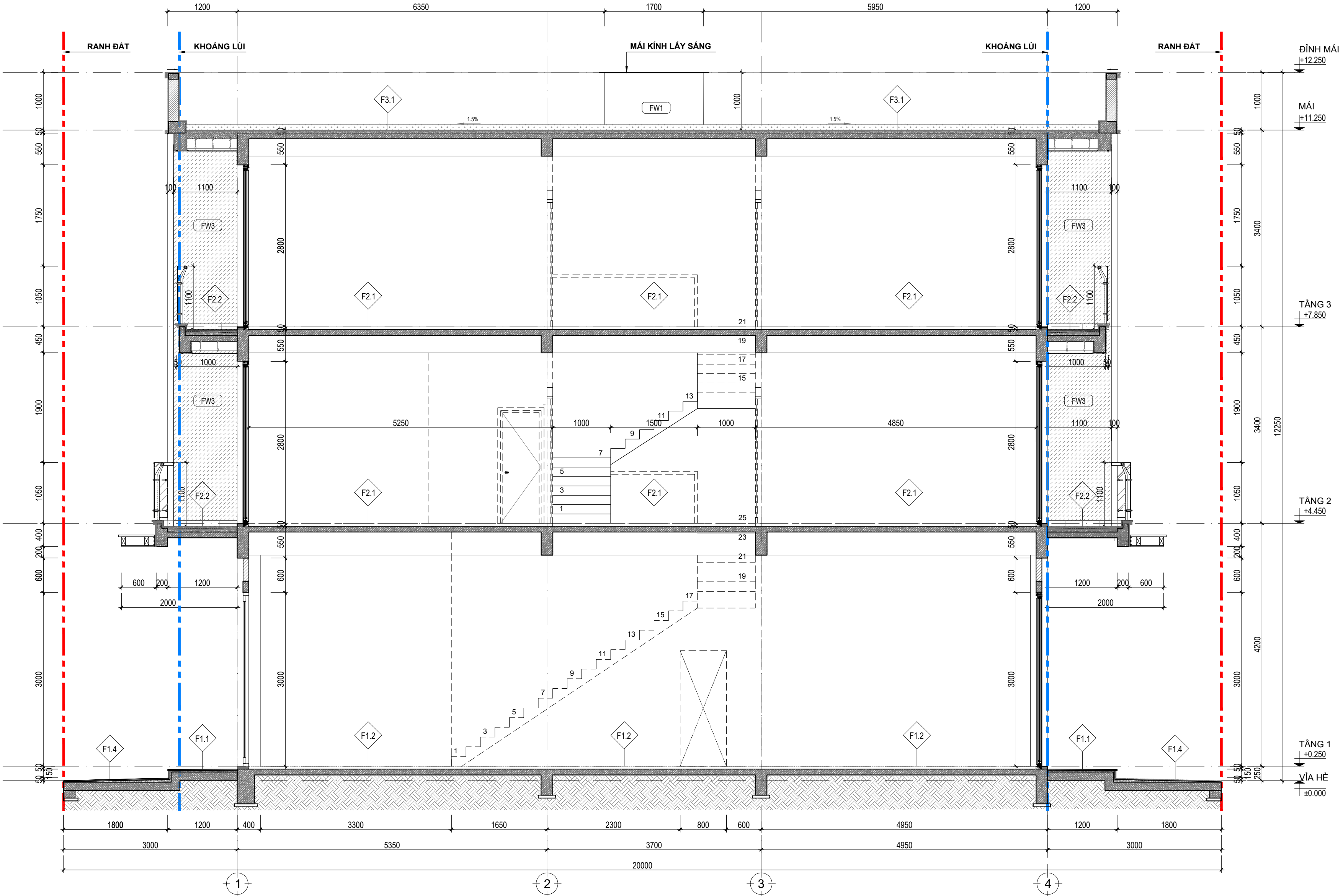
MẶT CẮT B-B _ TL:1/50
