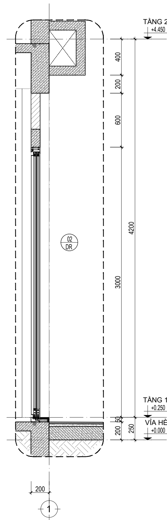
M. CẮT TRÍCH ĐOẠN 2-2_TL:1/25
