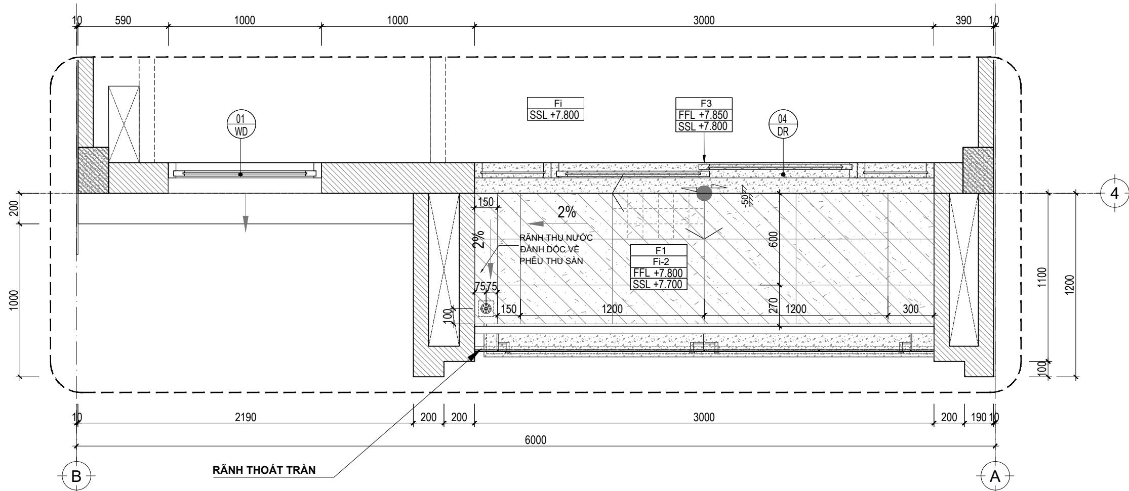
MẶT BẰNG TRÍCH ĐOẠN B-A - TẦNG 3_TL:1/25
