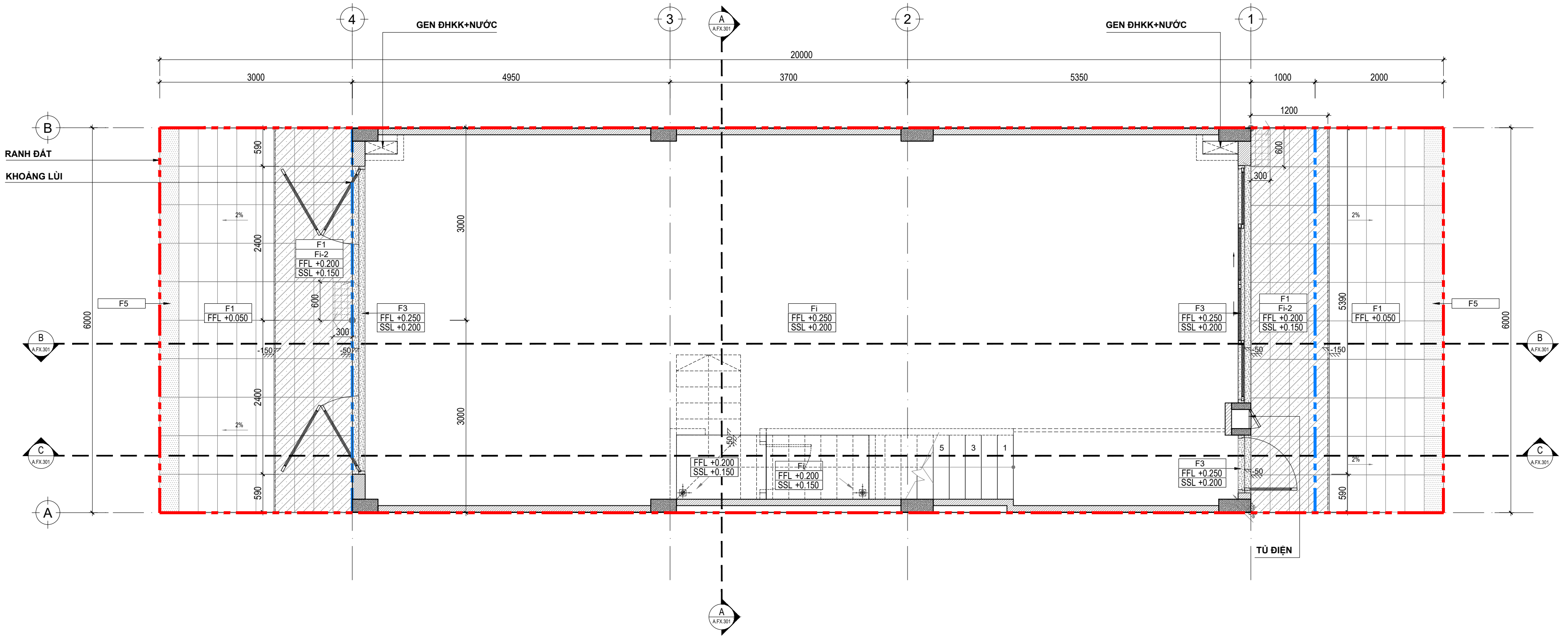
MẶT BẰNG HOÀN THIỆN SÀN TẦNG 1 _ TL:1/50
