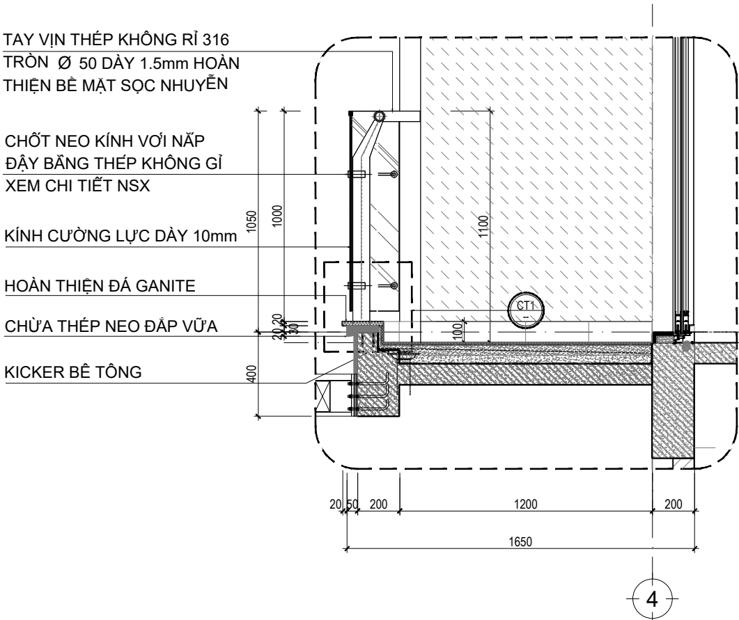
MC 1-1 BAN CÔNG TẦNG 2_TL:1/25
