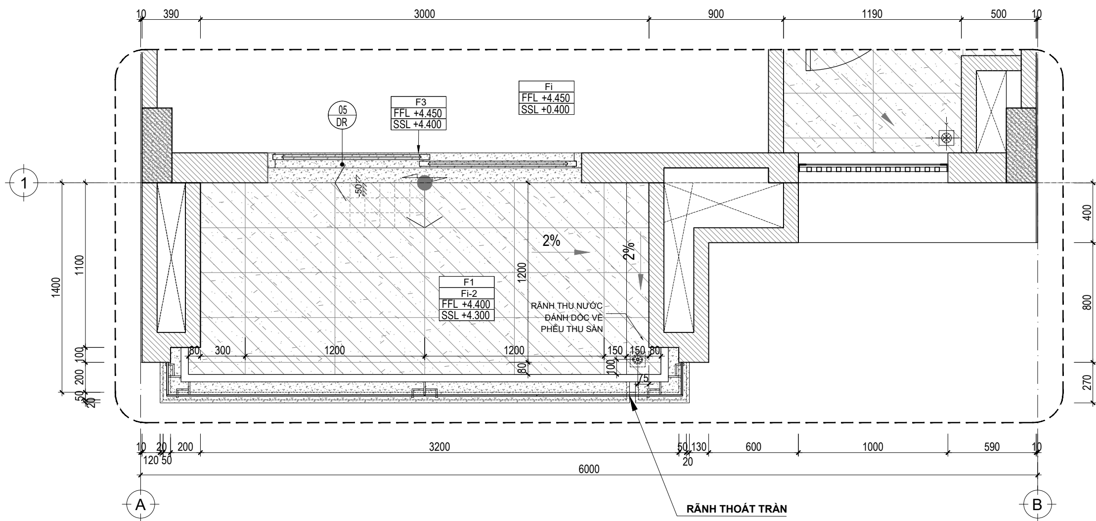
MẶT BẰNG TRÍCH ĐOẠN A-B - TẦNG 2_TL:1/25
