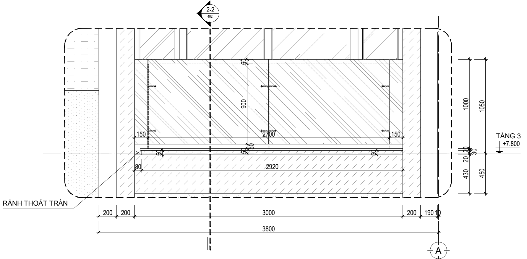
MẶT ĐỨNG BAN CÔNG TẦNG 3 ĐIỂN HÌNH_TL:1/25
