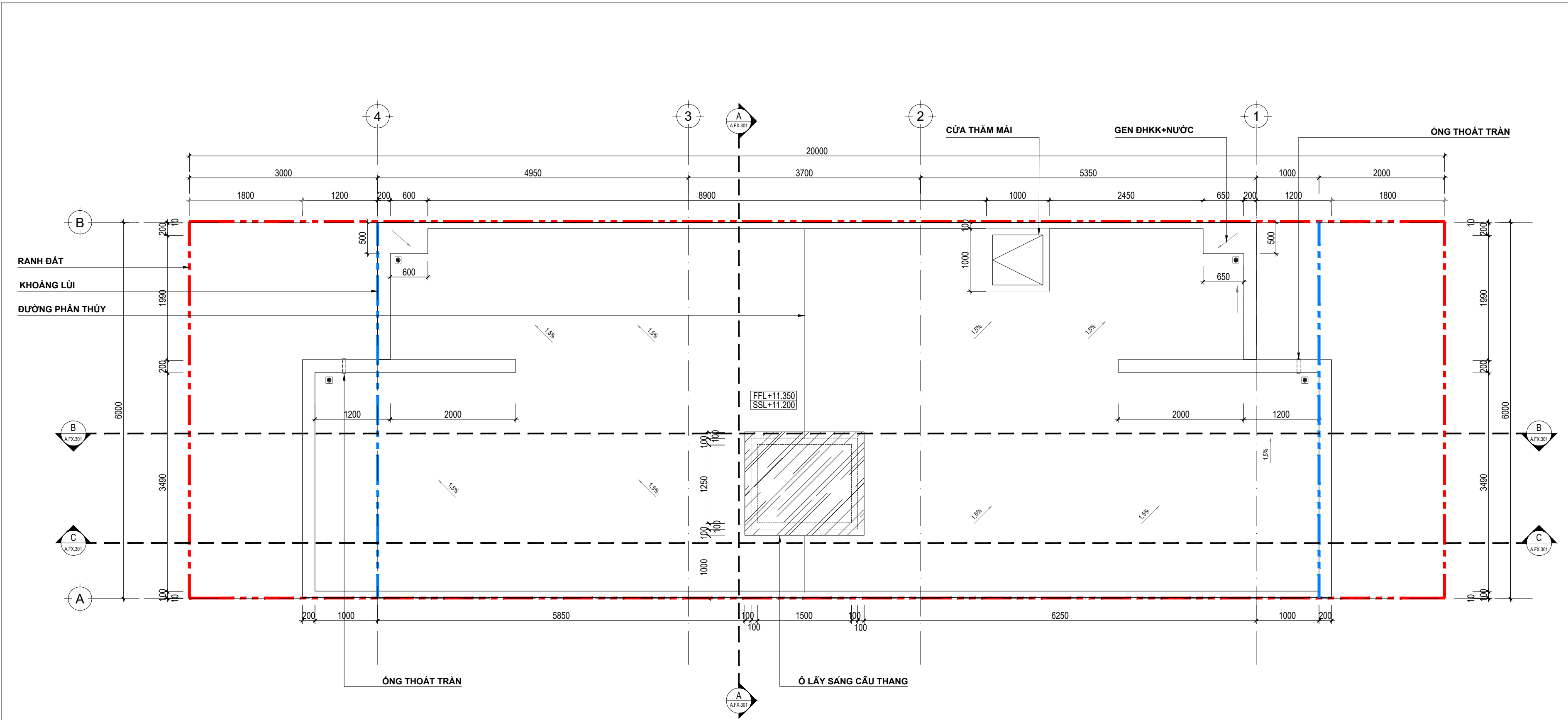
MẶT BẰNG KÍCH THƯỚC TẦNG MÁI _ TL:1/50
