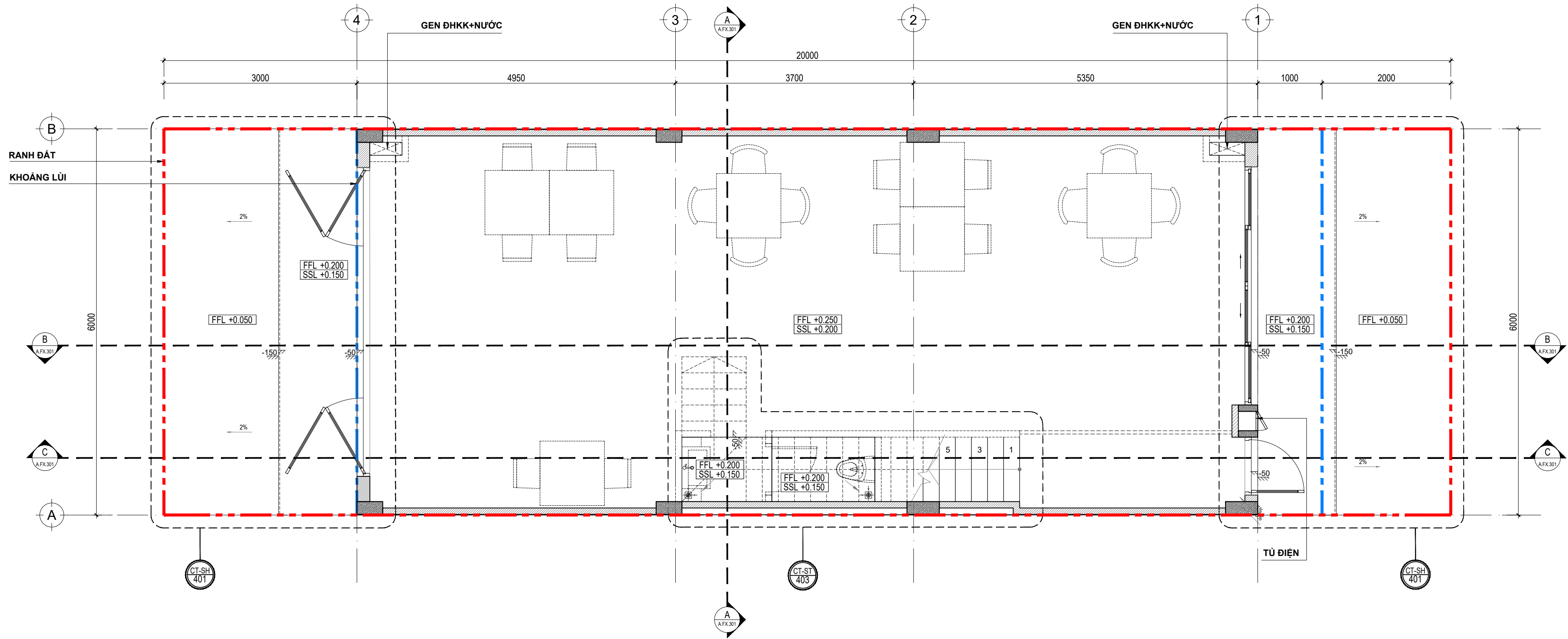
MẶT BẰNG KIẾN TRÚC TẦNG 1 _ TL:1/50
