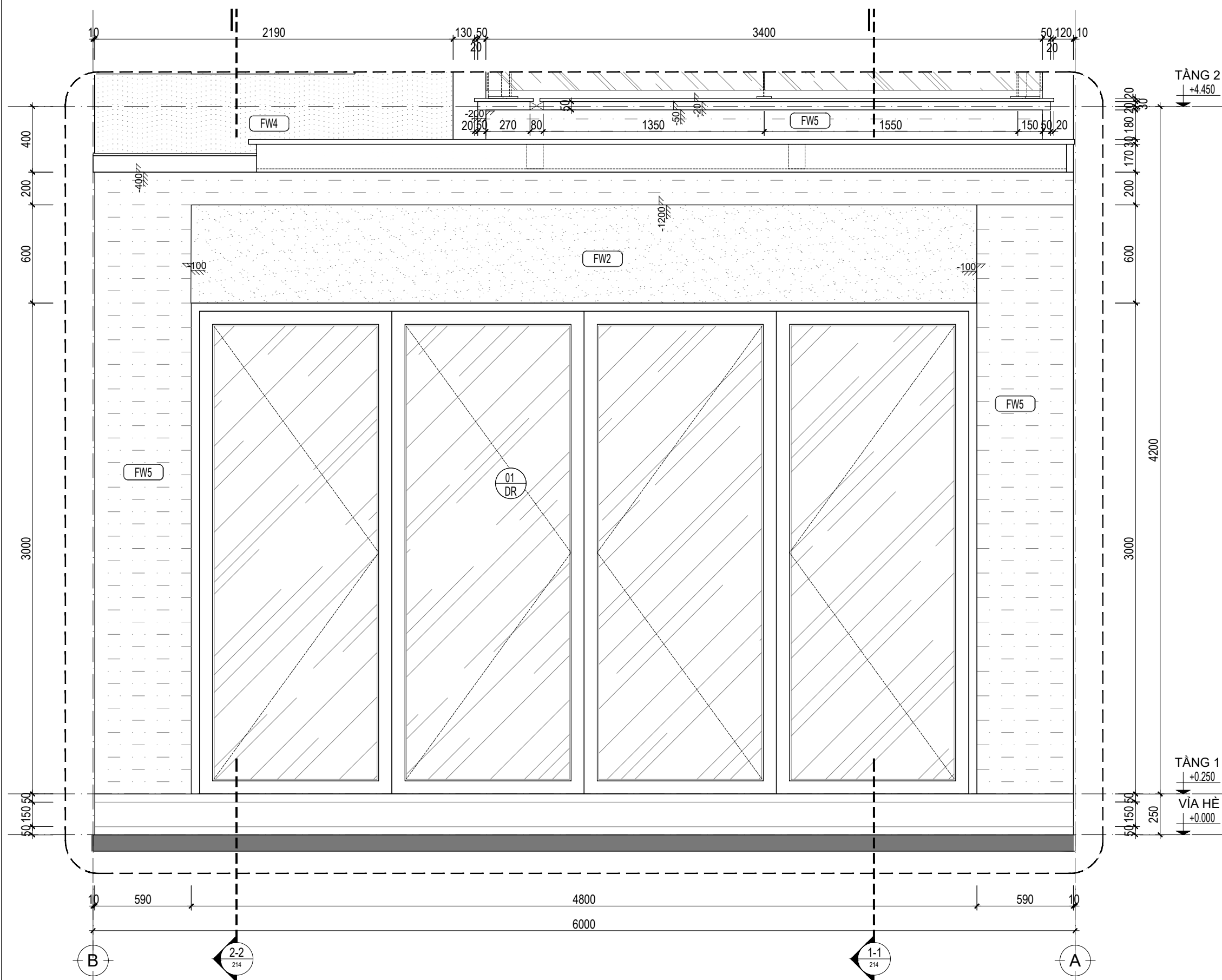
MẶT ĐƯNG TRÍCH ĐOẠN B-A - TẦNG 1_TL:1/25
