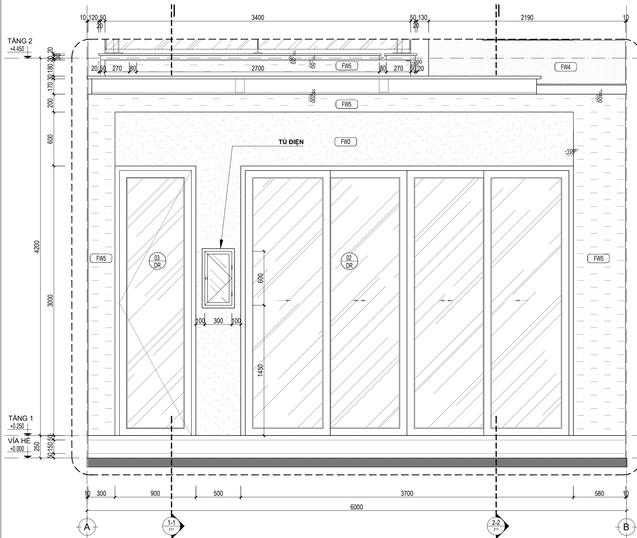
MẶT ĐỨNG TRÍCH ĐOẠN A-B - TẦNG 1_TL:1/25
