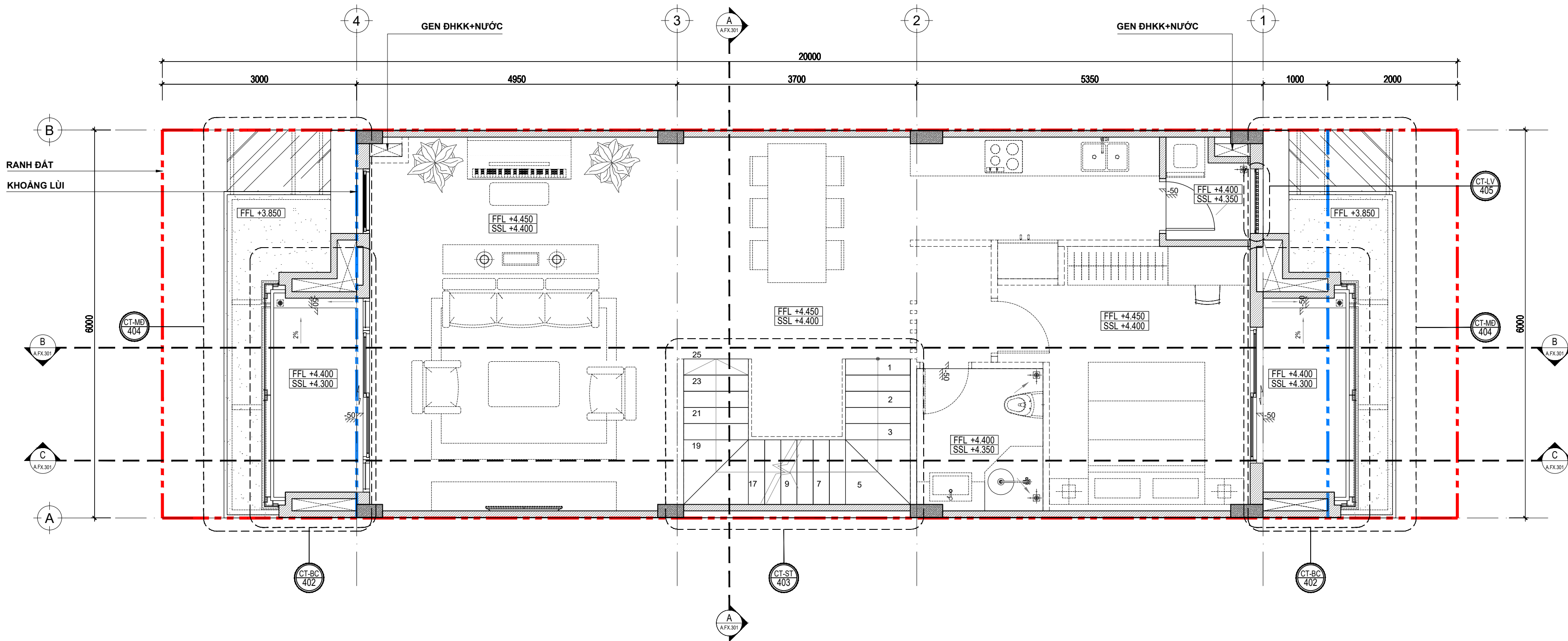
MẶT BẰNG KIẾN TRÚC TẦNG 2 _ TL:1/50
