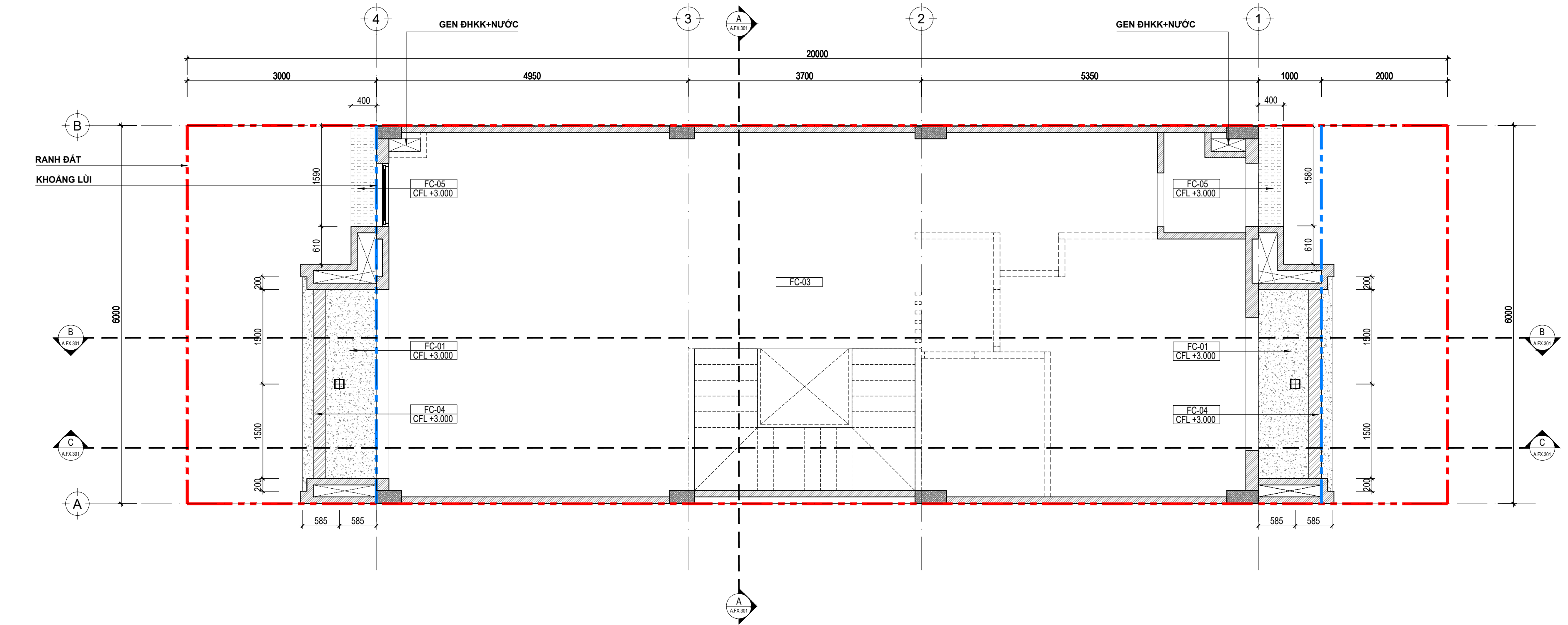
MẶT BẰNG TRẦN TẦNG 2_ TL:1/50
