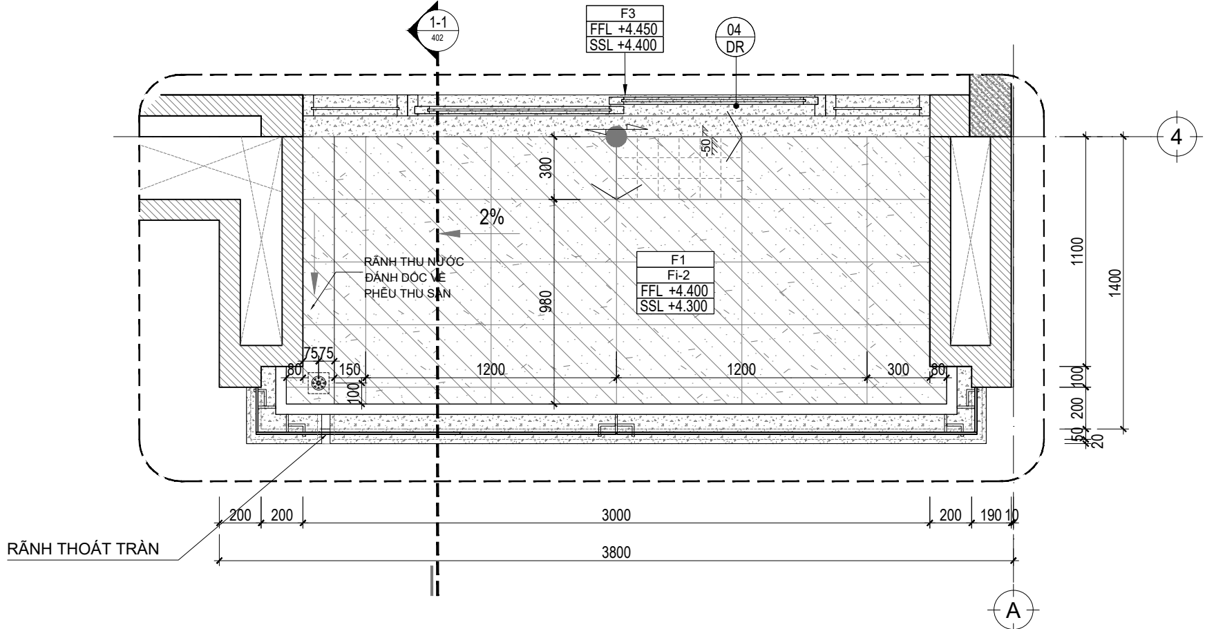
MẶT BẰNG BAN CÔNG TẦNG 2 ĐIỂN HÌNH_TL:1/25
