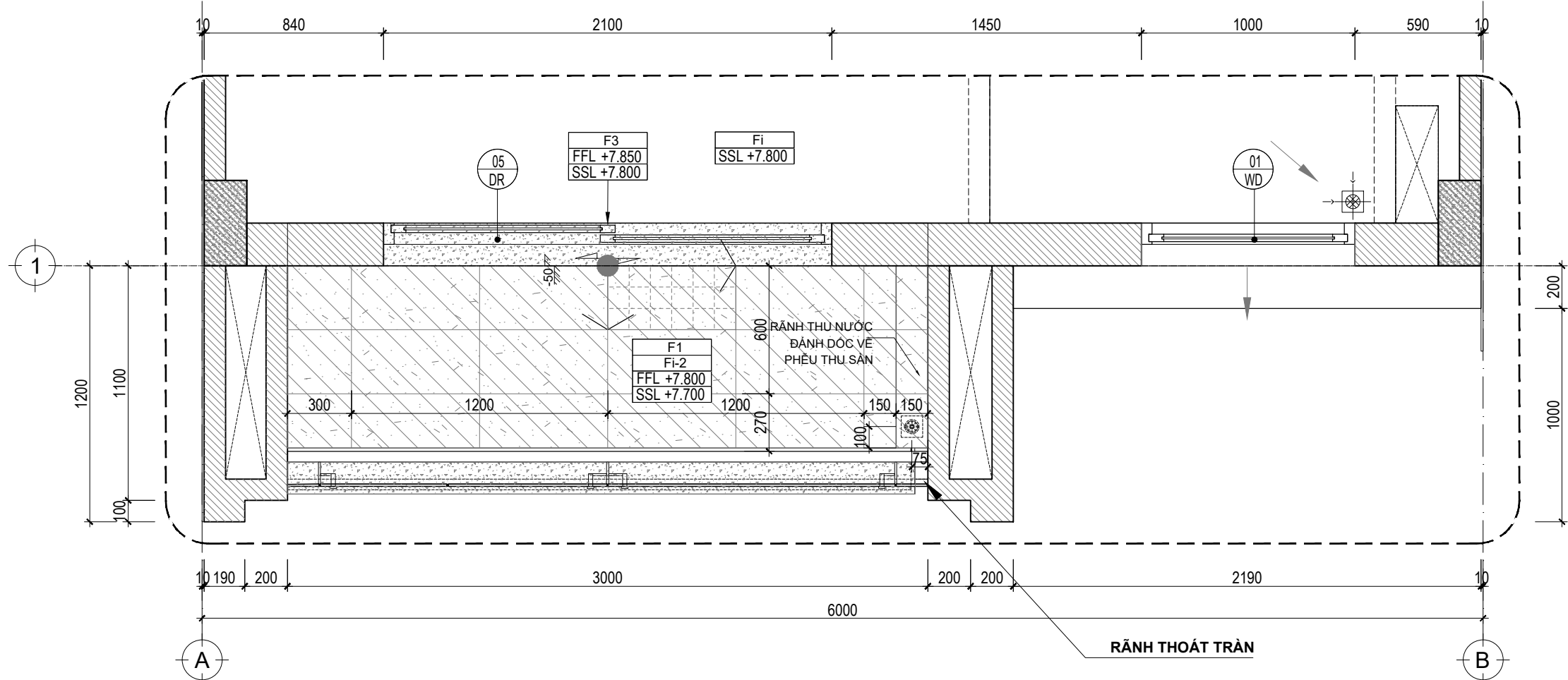
MẶT BẰNG TRÍCH ĐOẠN A-B - TẦNG 3_TL:1/25
