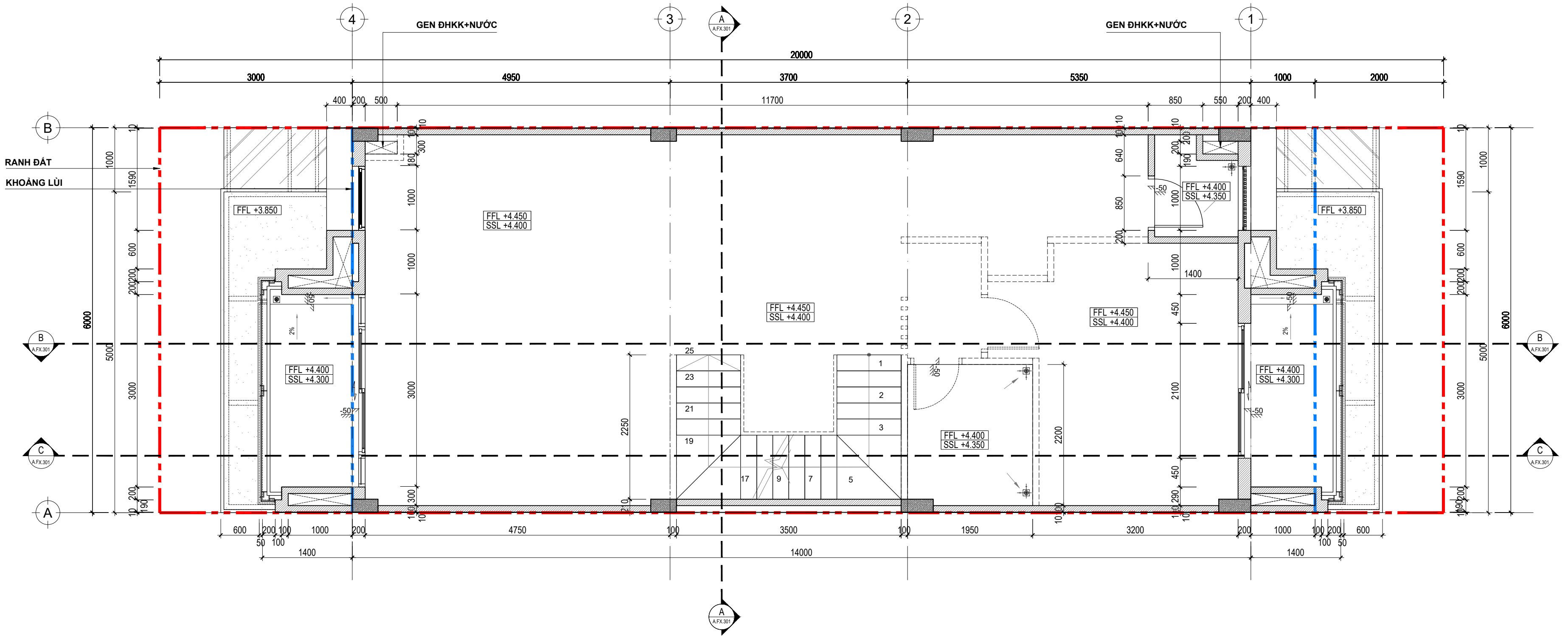
MẶT BẰNG KÍCH THƯỚC TẦNG 2_ TL:1/50
