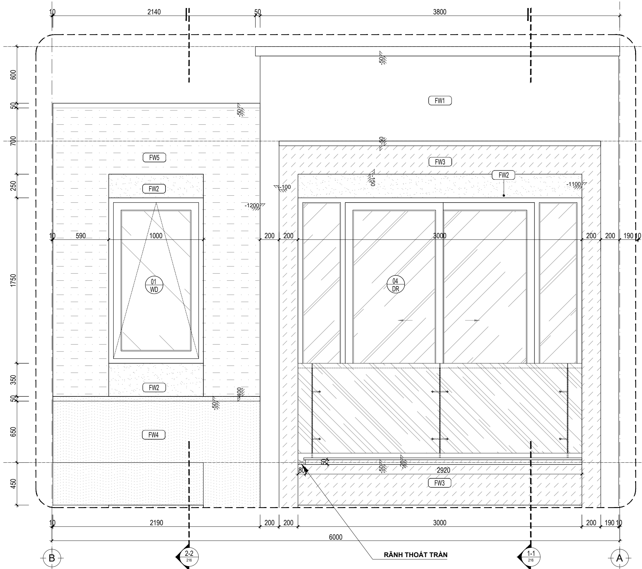
MẶT ĐỨNG TRÍCH ĐOẠN B-A - TẦNG 3_TL:1/25
