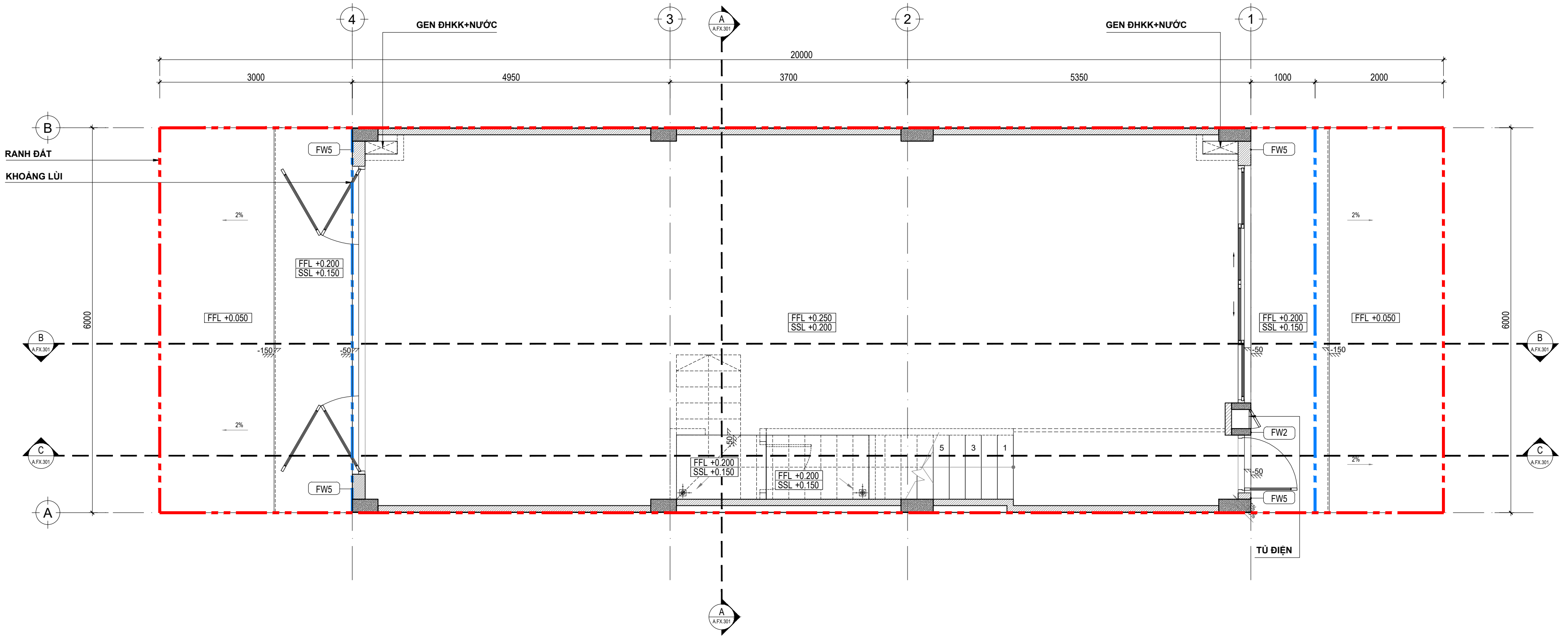
MẶT BẰNG HOÀN THIỆN TƯỜNG TẦNG 1 _ TL:1/50
