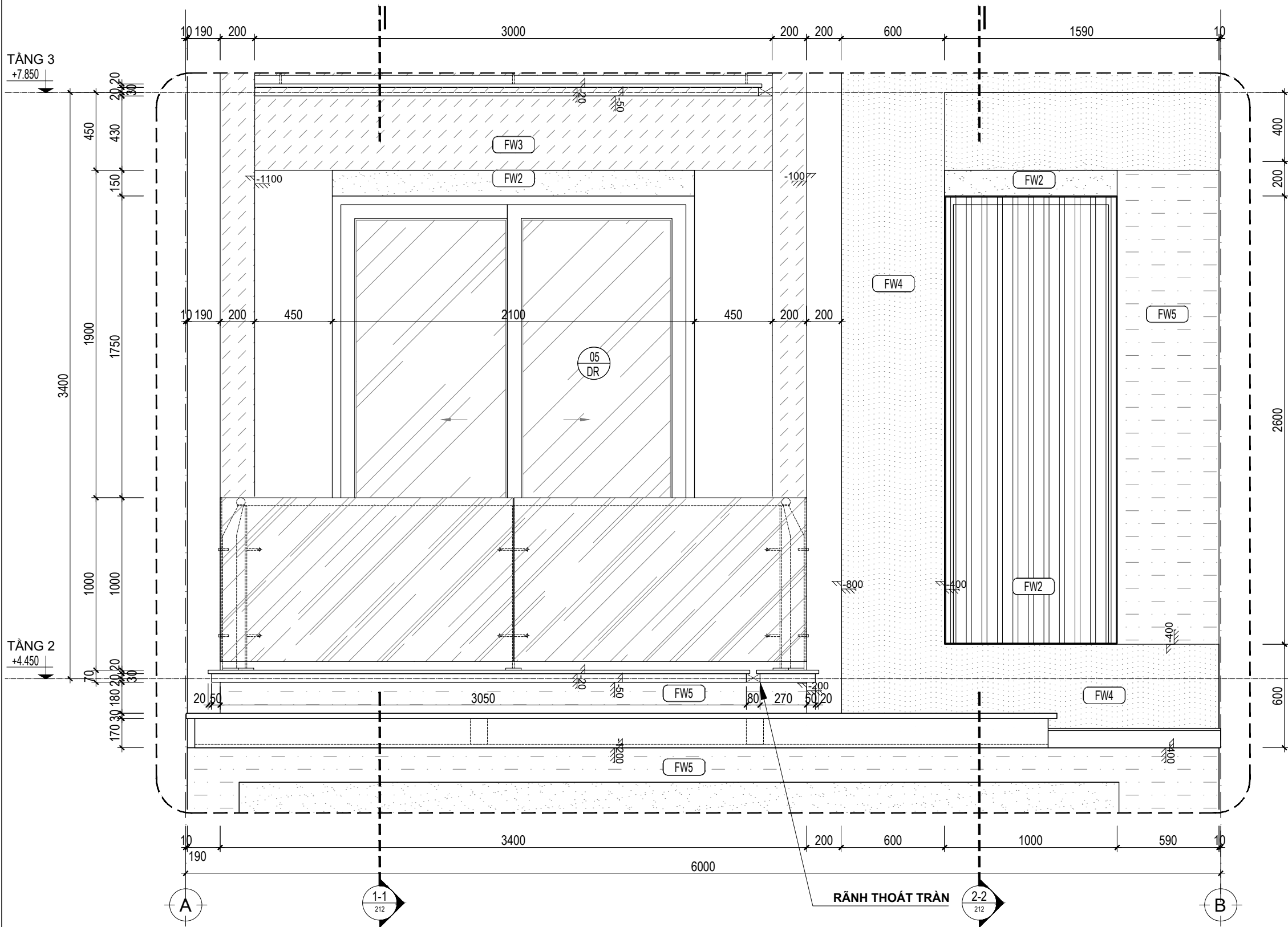
MẶT ĐƯNG TRÍCH ĐOẠN A-B - TẦNG 2_TL:1/25
