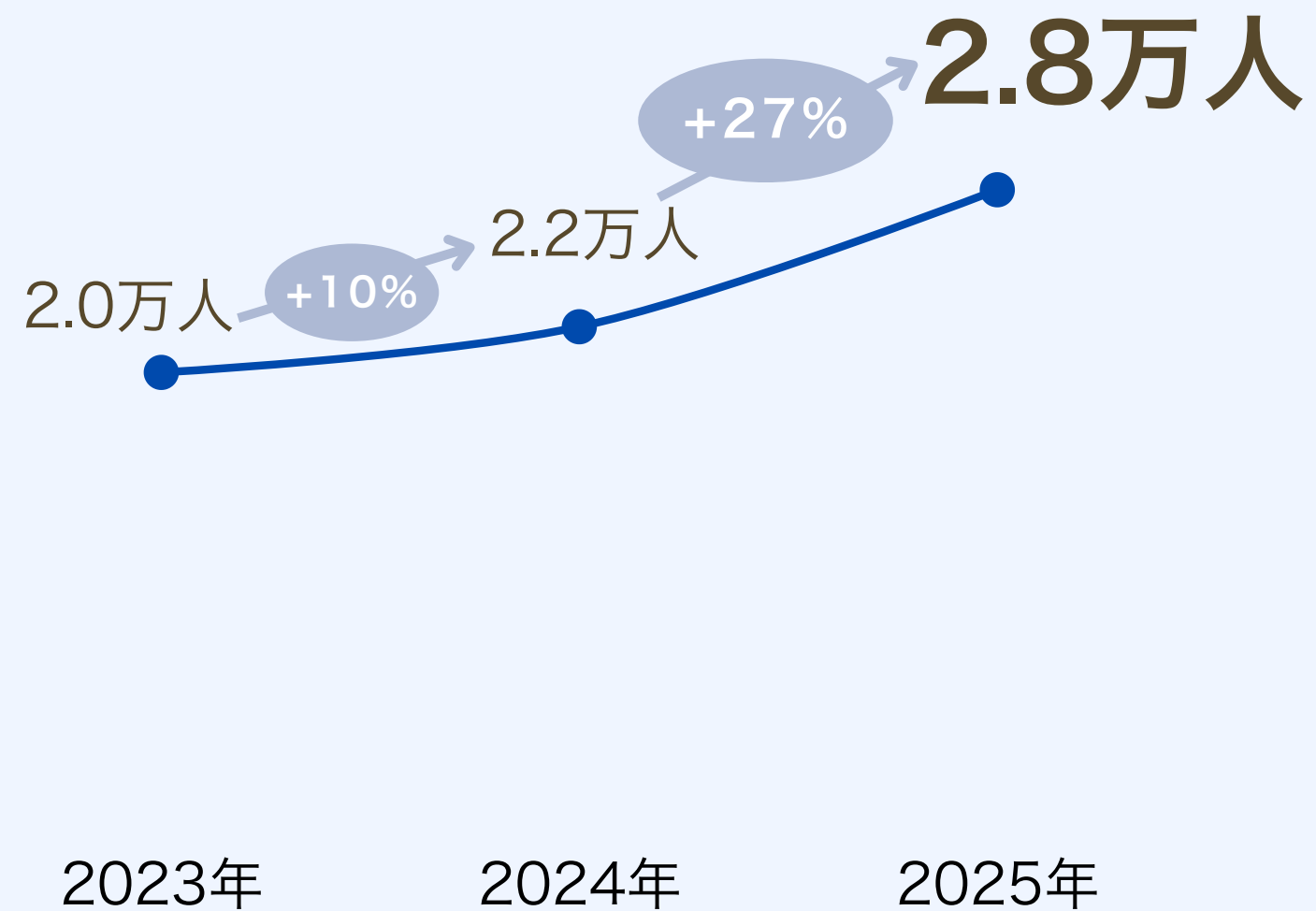
IBJ成婚者数の推移
