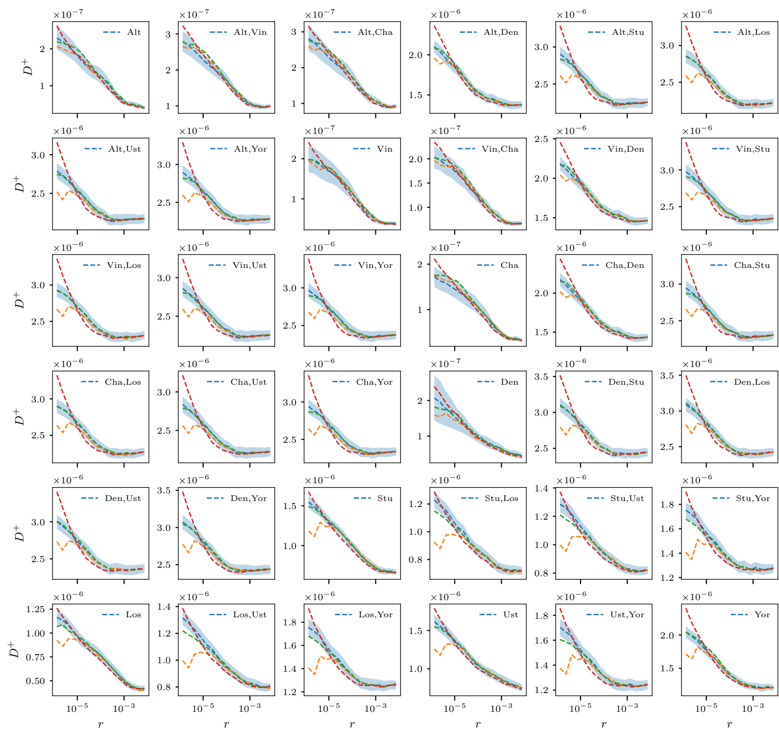
— Bhérier map - - HapMap map - - Omni YRI map - - Pyhro YRI map
