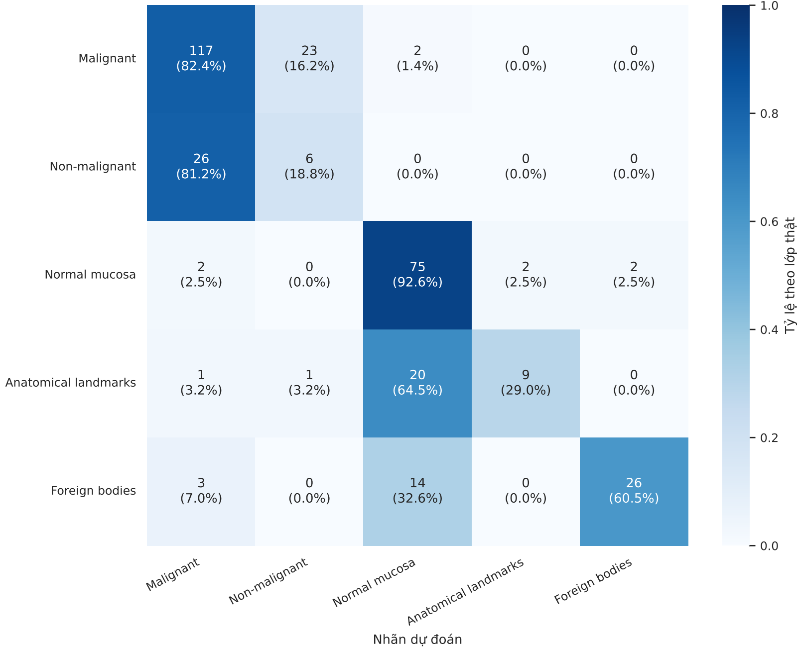
Ma trận nhầm lẫn 5 lớp (n = 329 ảnh test)
