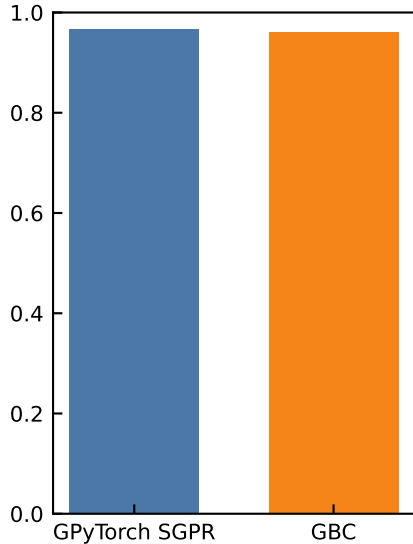
Test ROC-AUC
