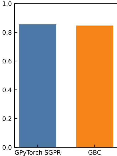
Test F1
