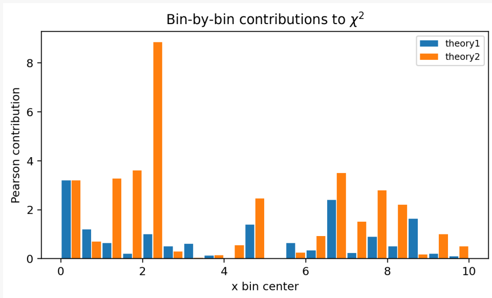
各区间对 Pearson \chi^2 的贡献; theory2 在高 x 区间贡献明显偏大。
