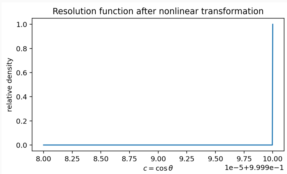
单支 x \geq 0 情形下，非线性变换后 c = \cos\theta 分辨率函数的示例。
