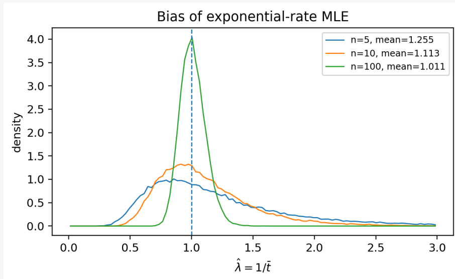
\hat{\lambda} = 1/\bar{\tau} 的模拟分布；小样本时右偏明显，且均值高于真值。
