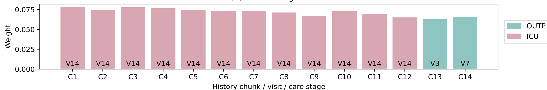
(d) Visit importance
