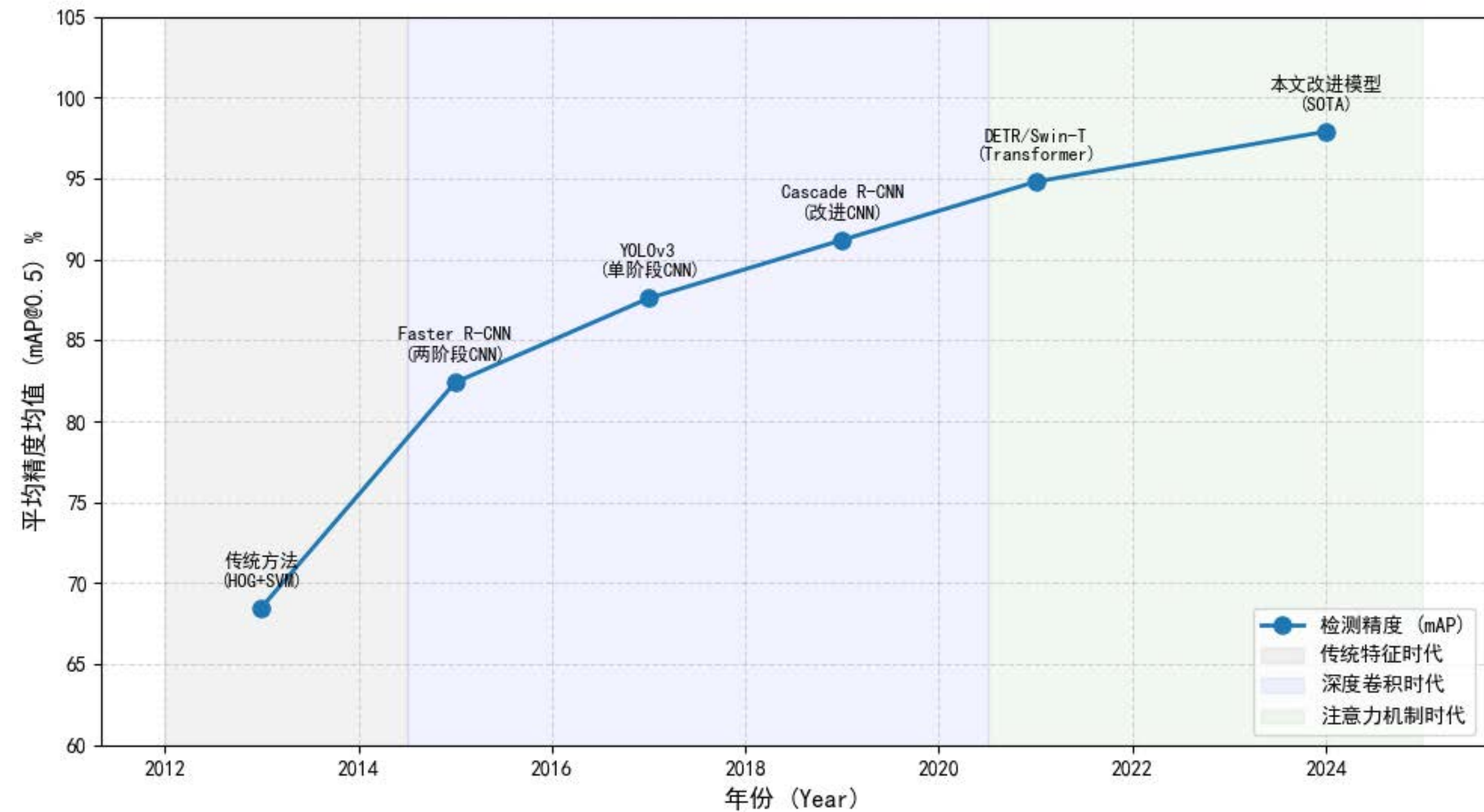
绝缘子缺陷检测模型性能演进趋势
