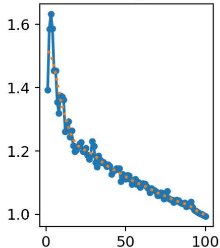
val/box_loss
