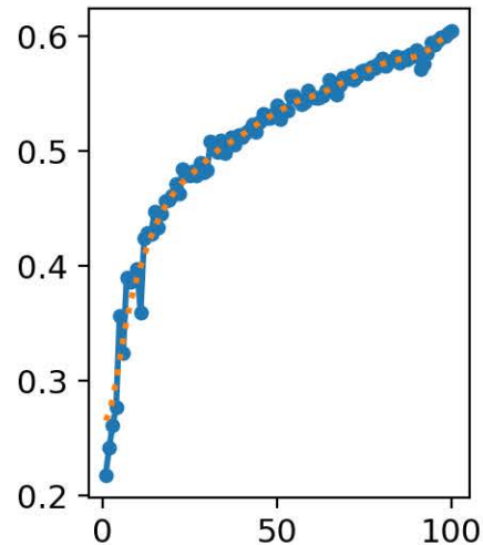
metrics/mAP50-95(B)
