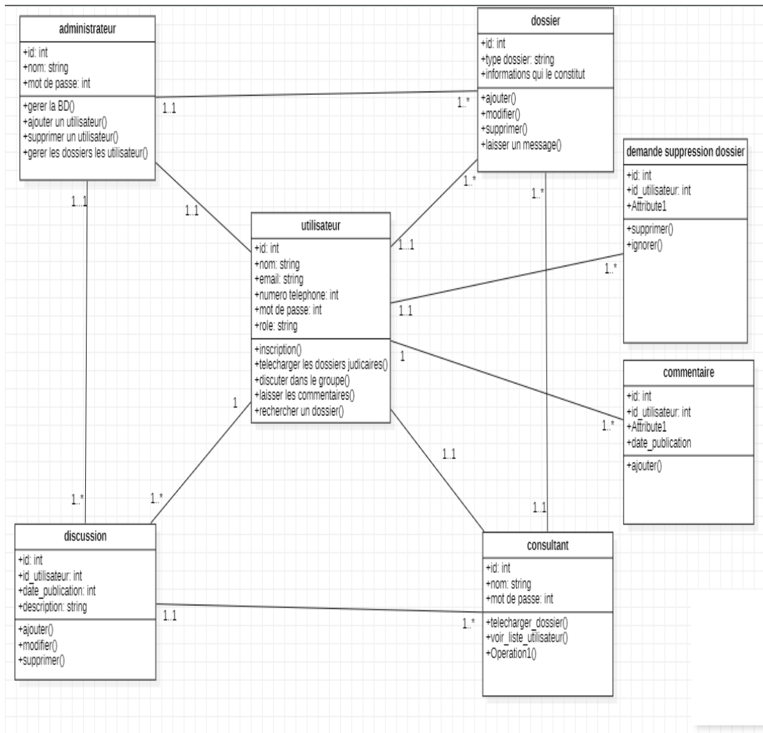
Figure 11:Diagramme de classe récapitulatif
