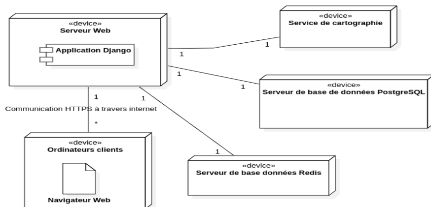
Figure 13: Diagramme de déploiement
