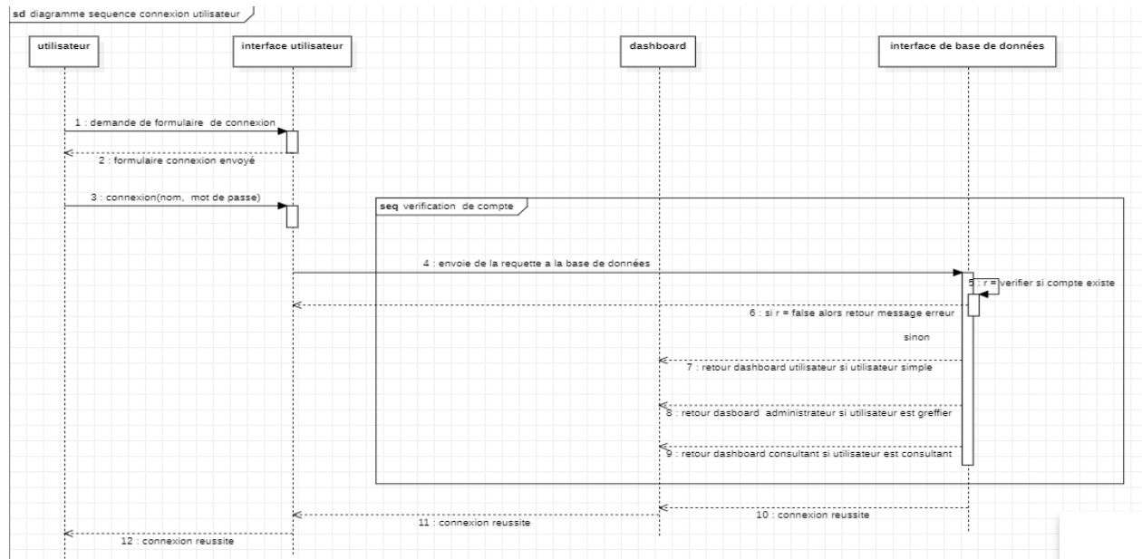
Figure 9:Diagramme de séquence connexion
