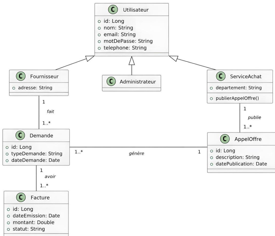
Figure 2.4 : Vue synthétique des entités métier principales.
