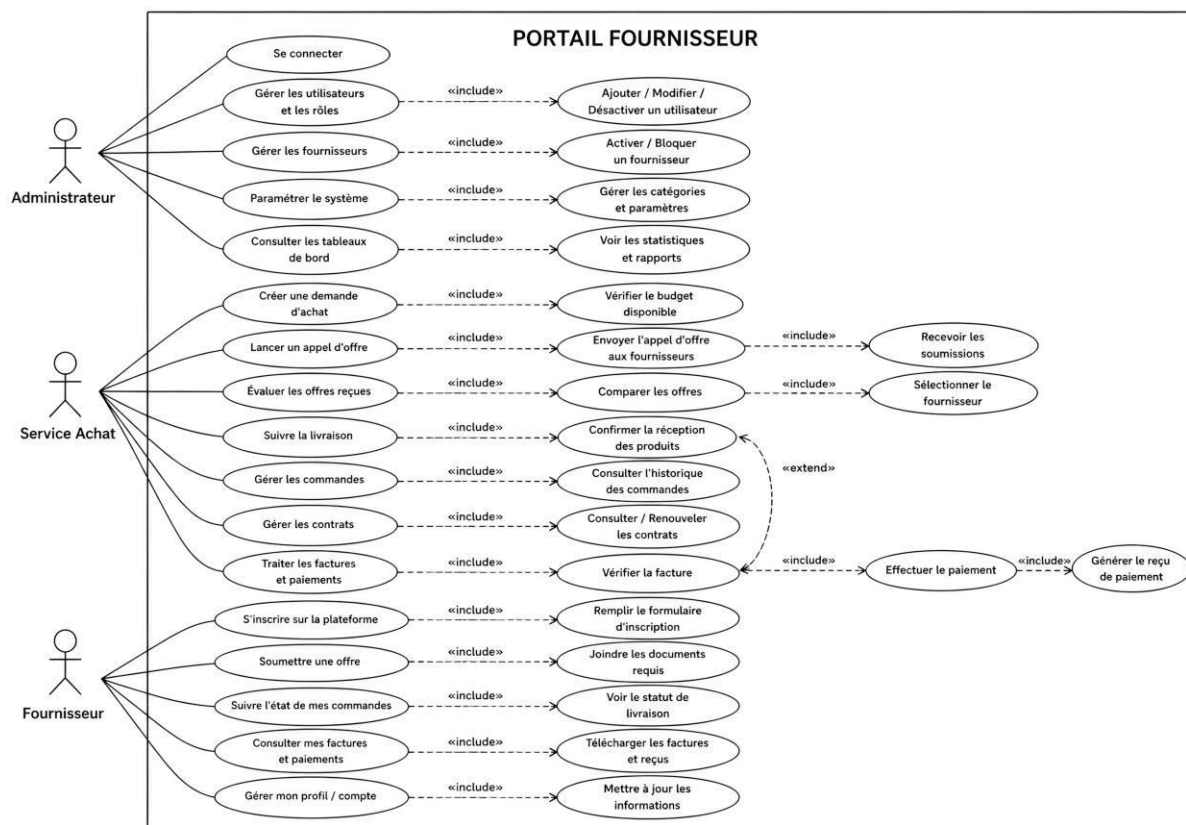
Figure 2.3 : Principaux cas d'utilisation selon les trois profils du système.
