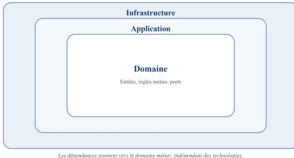
Figure 2.2 : Organisation du back-end selon la Clean Architecture.
