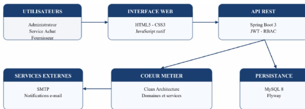
Figure 2.1 : Architecture générale du Portail Fournisseur.
