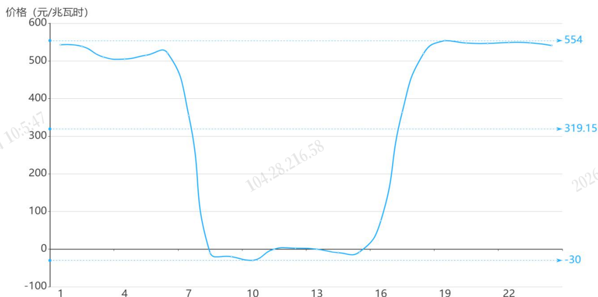
图 2 9 月 3 日日前市场用电侧价格
