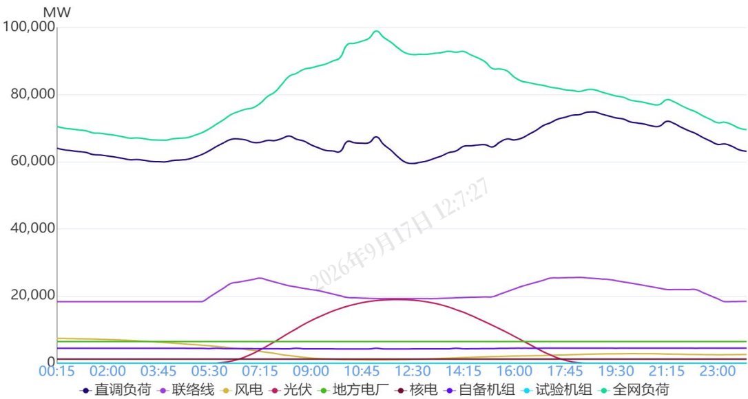
图 1 9月13日负荷及电源出力预测情况
