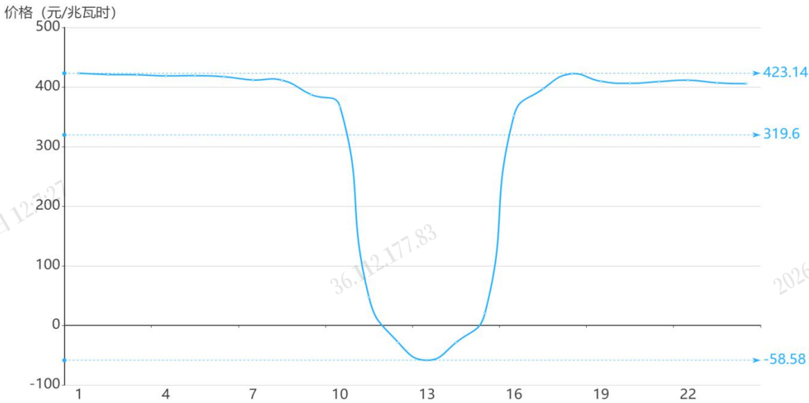
图 3 9 月 12 日实时市场用电侧价格
