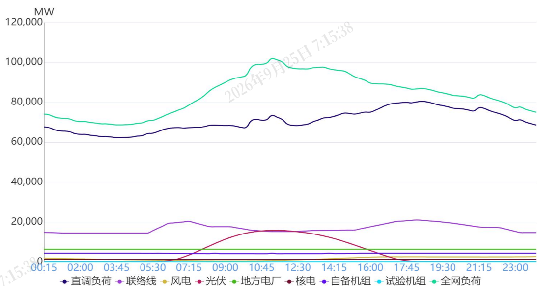
图1 9月20日负荷及电源出力预测情况
