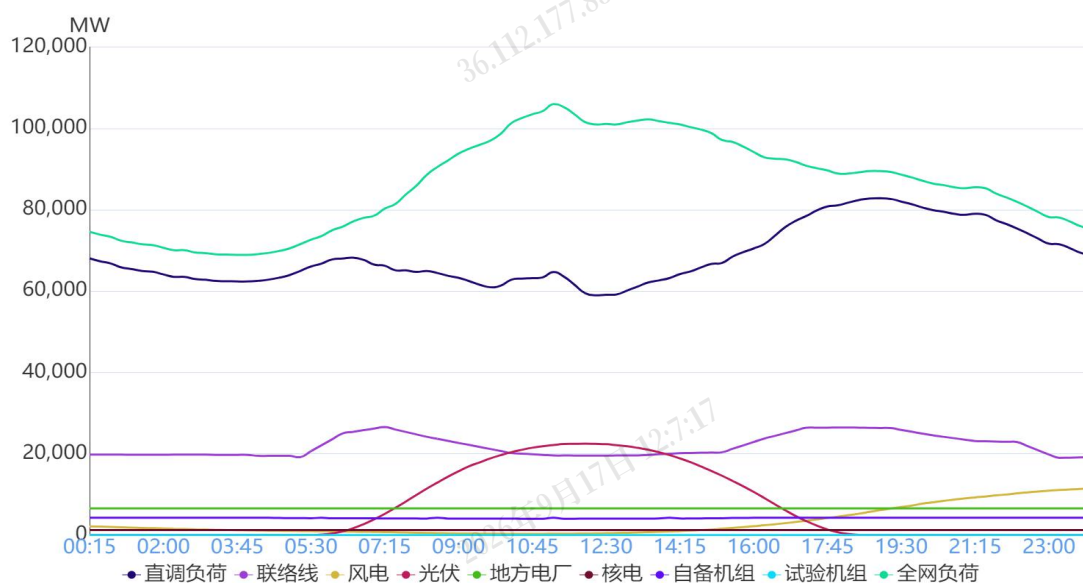
图 1 9月7日负荷及电源出力预测情况
