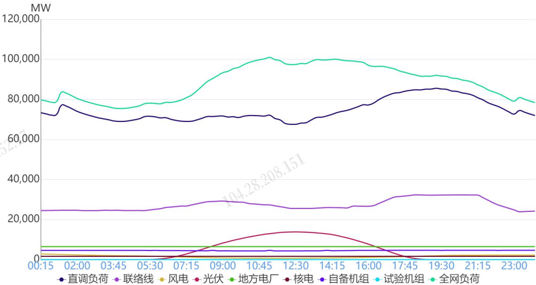
图 1 8月29日负荷及电源出力预测情况
