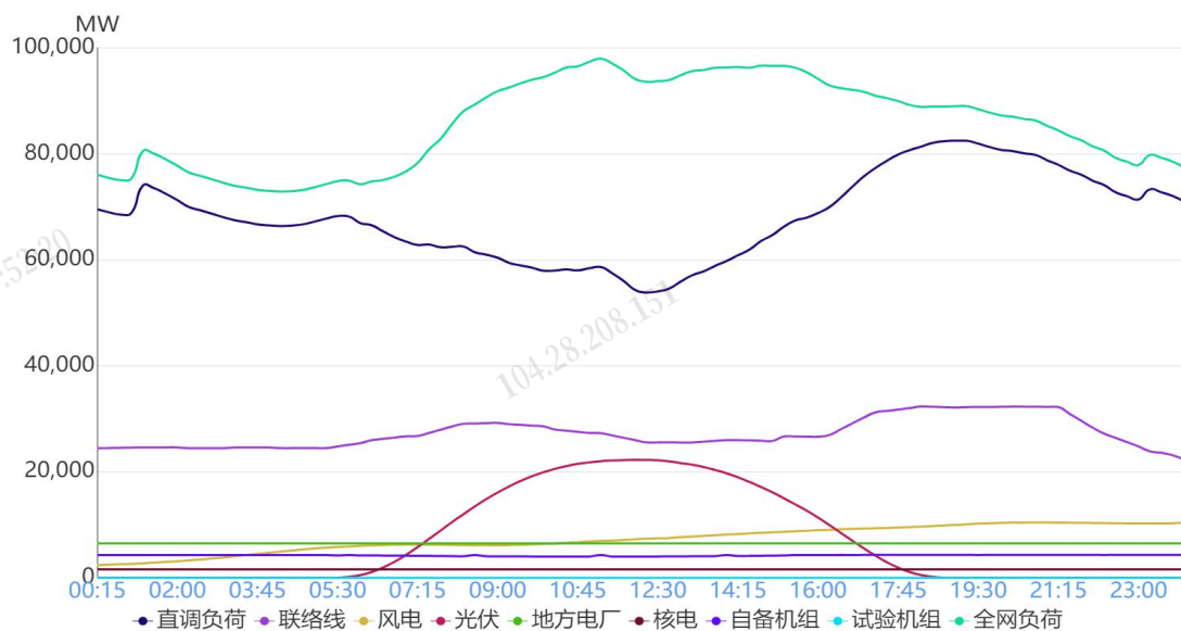
图1 8月31日负荷及电源出力预测情况
