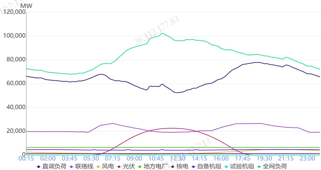
图 1 9 月 5 日负荷及电源出力预测情况
