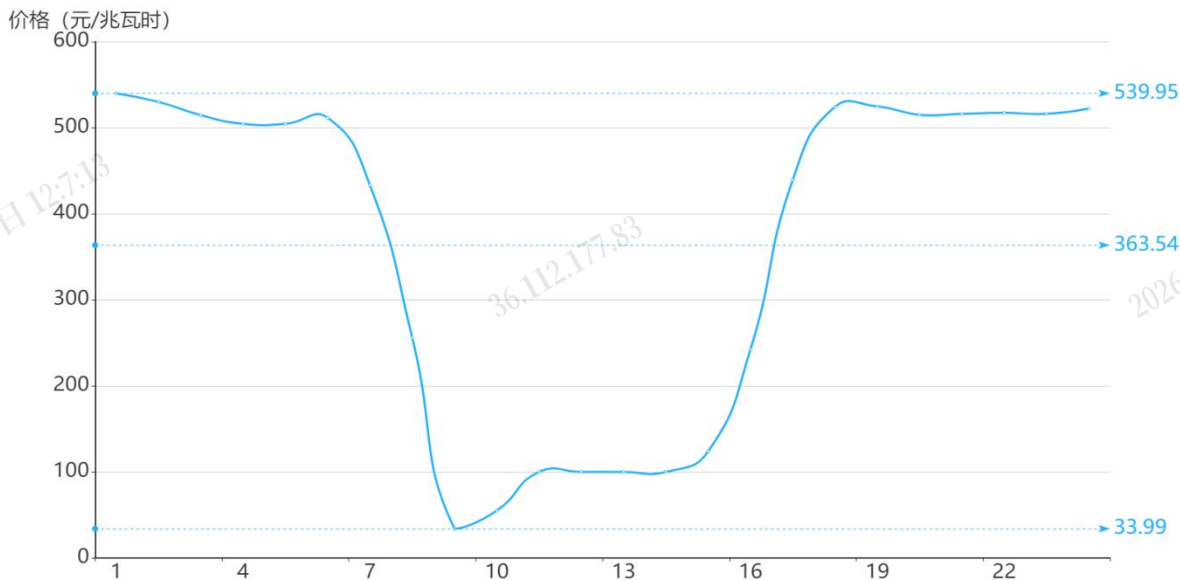
图2 9月5日日前市场用电侧价格
