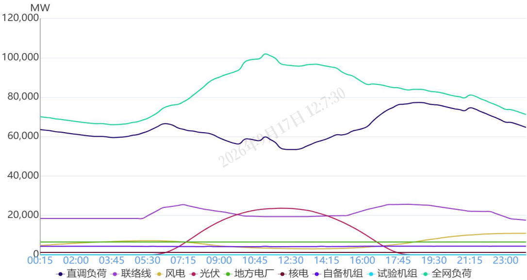
图 1 9月15日负荷及电源出力预测情况
