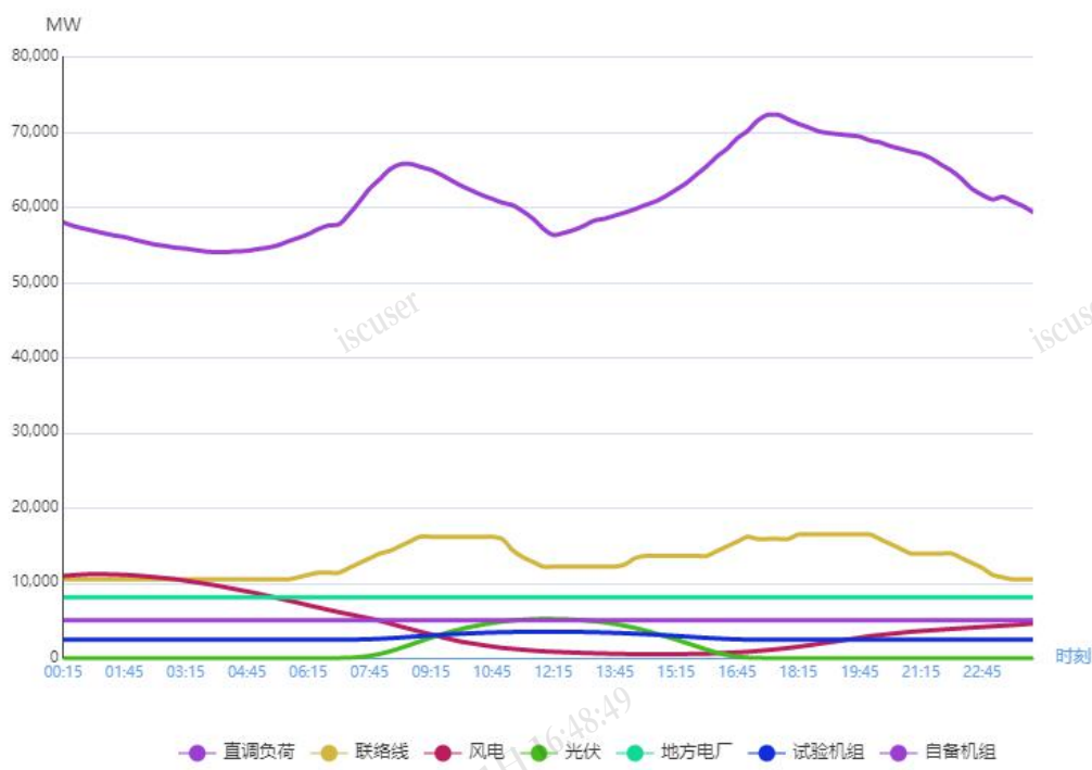
图 1 1 月 2 日负荷及电源出力预测情况
