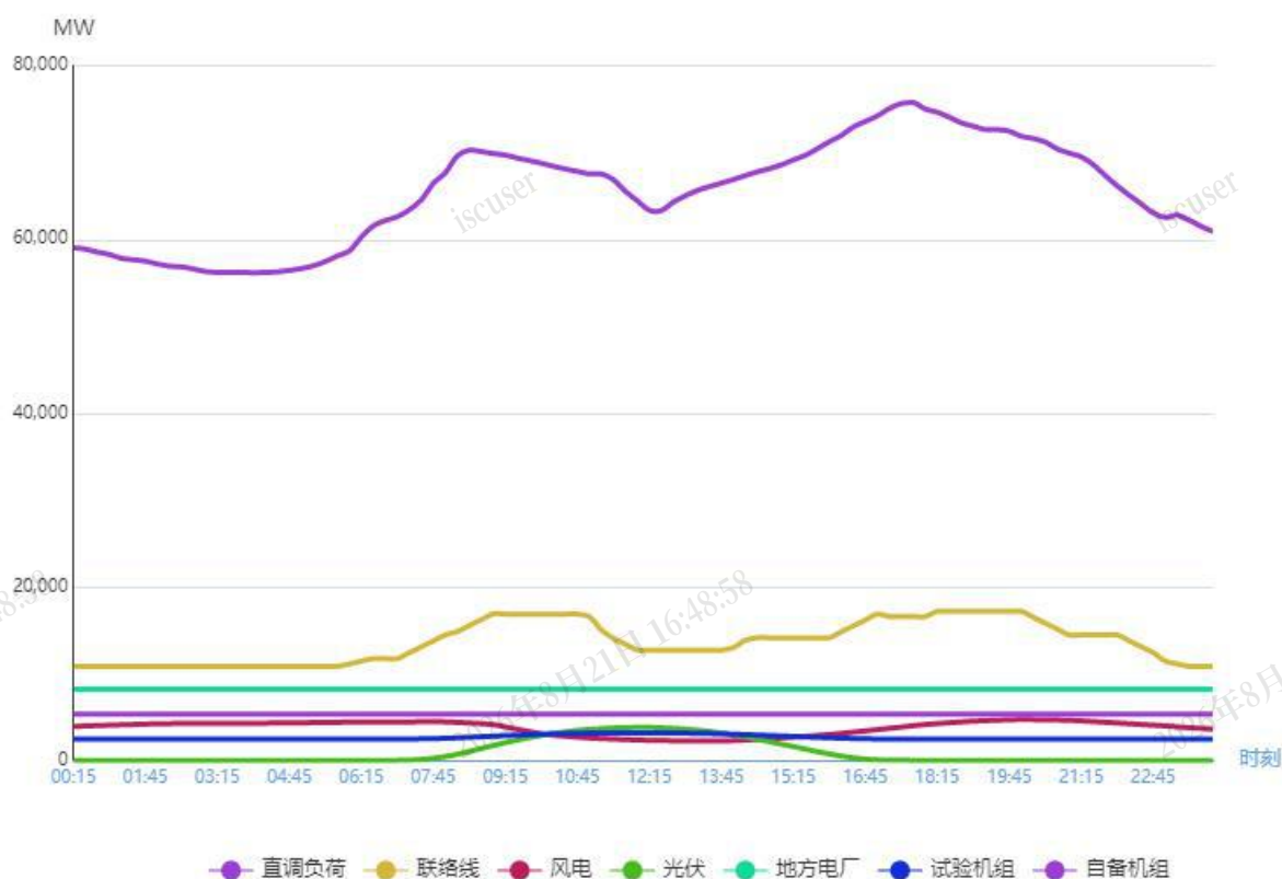
图 1 1月4日负荷及电源出力预测情况
