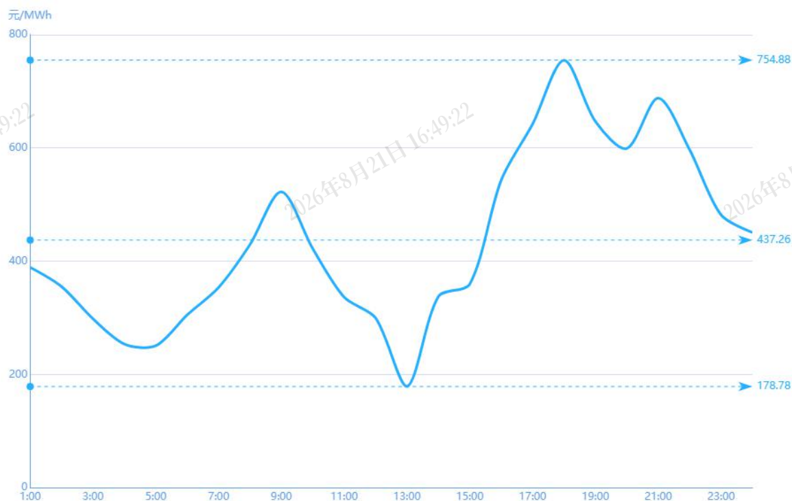
图 3 1 月 9 日实时市场用电侧价格
